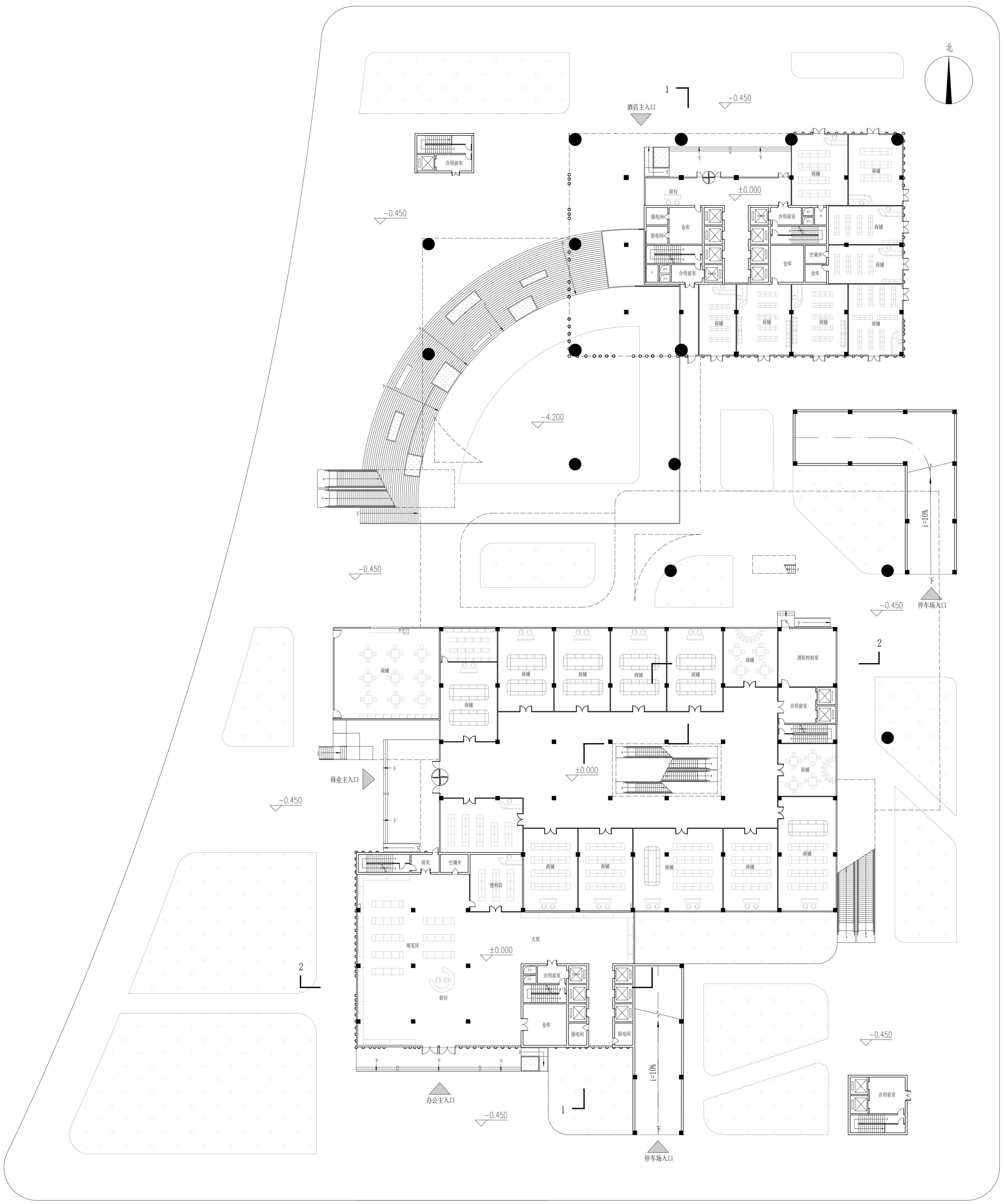
一层平面图 1:300
