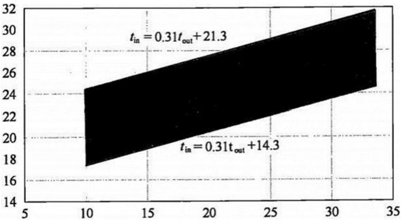
图 1 自然通风或复合通风建筑室内舒适温度范围
