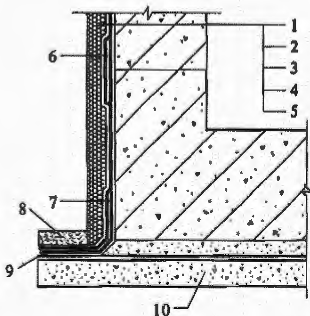
图 4.4.5-1 防水涂料外防外涂构造
