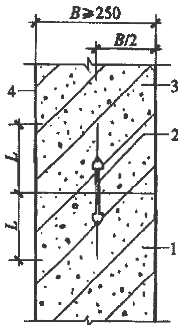
图 4.1.25-1 施工缝防水构造(一)
