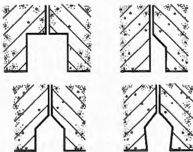
图 8.1.8 管片嵌缝槽断面构造形式
