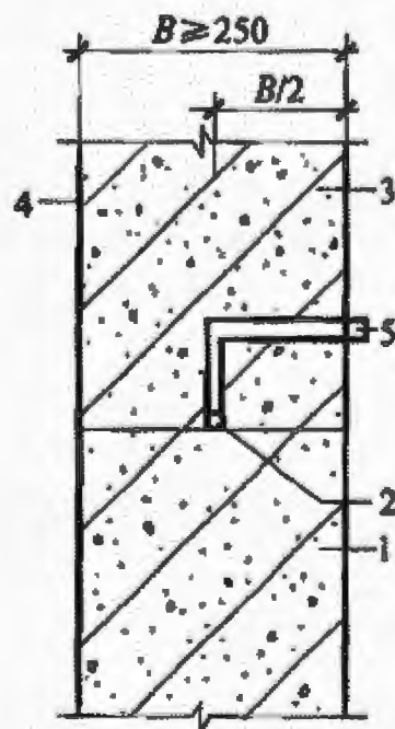
图 4.1.25-4 施工缝防水构造(四)
