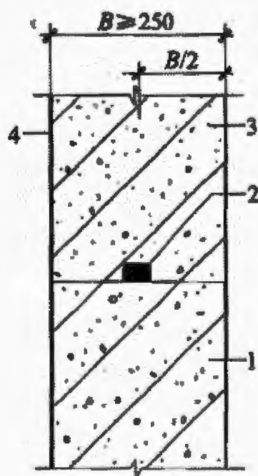
图 4.1.25-3 施工缝防水构造(三)
