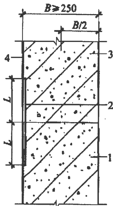
图 4.1.25-2 施工缝防水构造(二)
