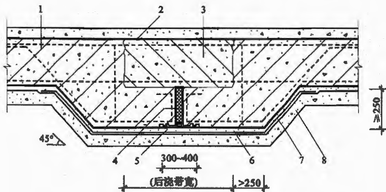
图 5.2.14 后浇带超前止水构造
