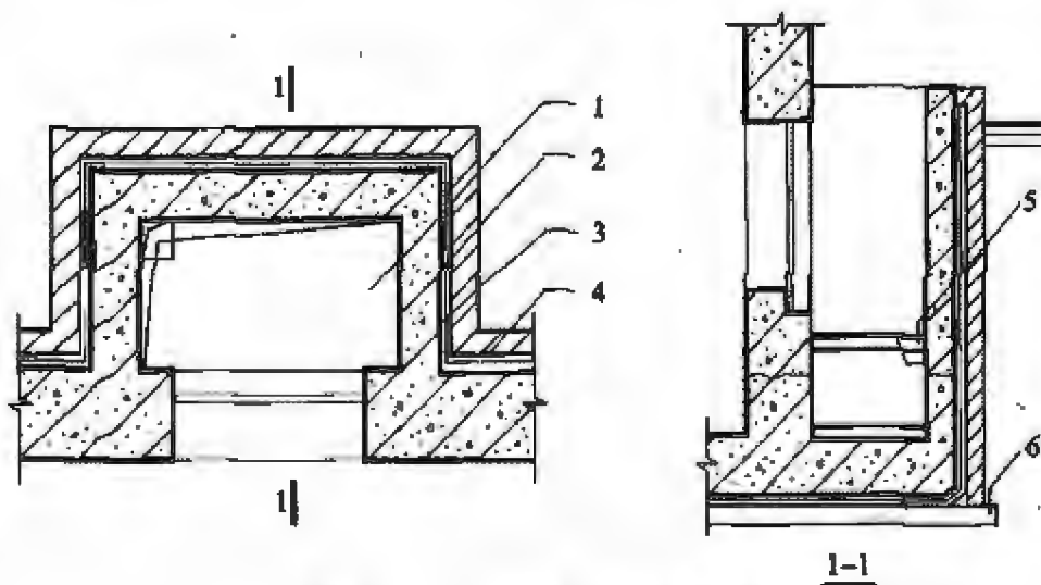
图 5.7.3 窗井防水构造
