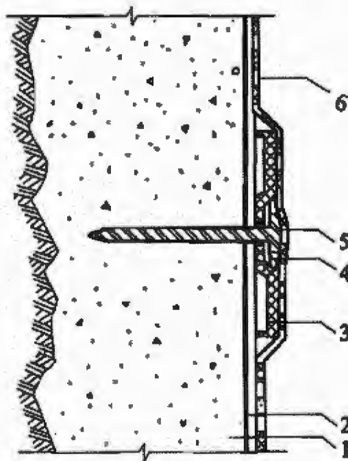
图 4.5.12 暗钉圈固定缓冲层
