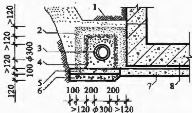
图 6.2.5-1 贴墙盲沟设置
