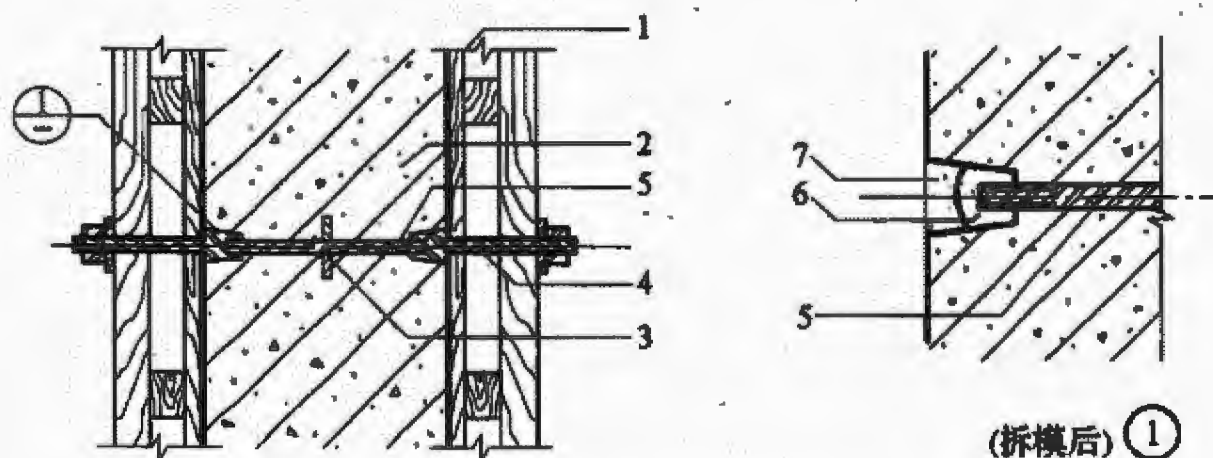
图 4.1.28 固定模板用螺栓的防水构造
