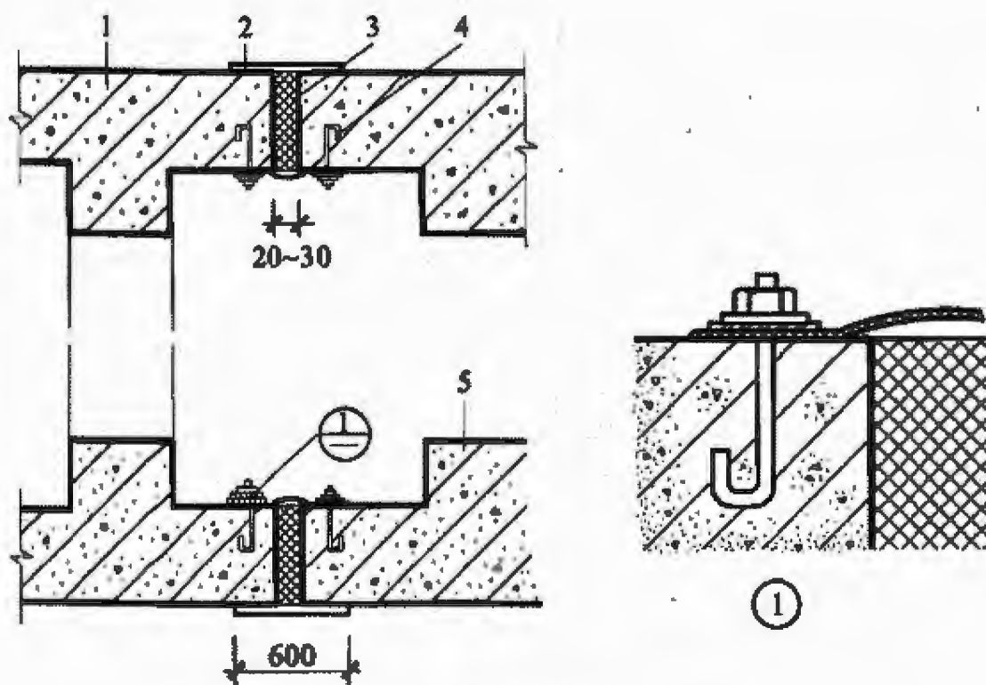
图 5.5.2-2 预留通道接头防水构造(二)
