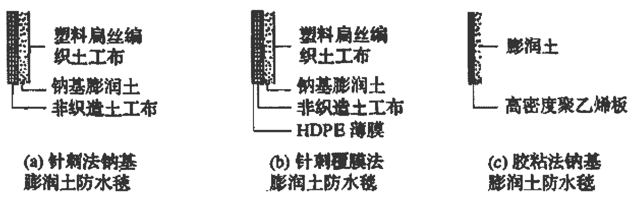
图 1 钠基膨润土防水毯
