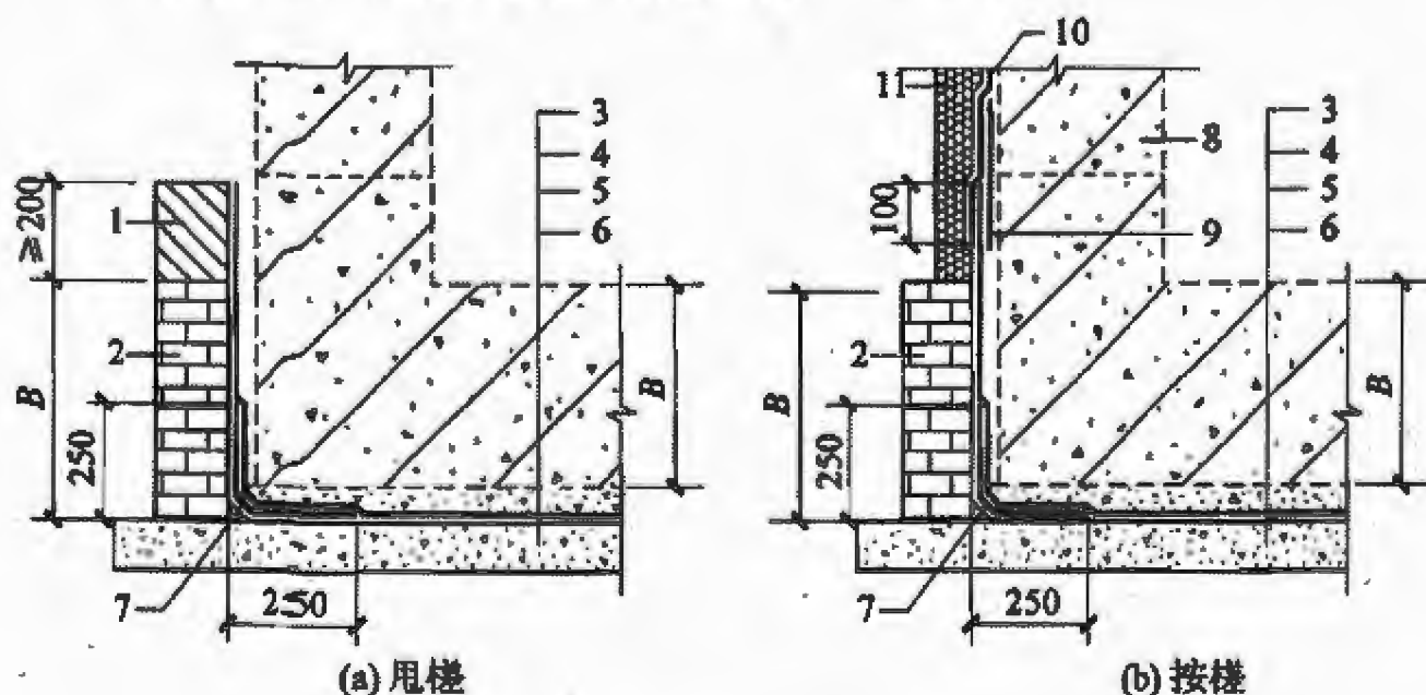
图4.3.23 卷材防水层甩槎、接槎构造
