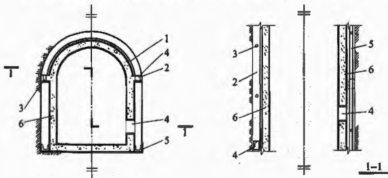
图 6.2.13 离壁式衬砌排水构造
