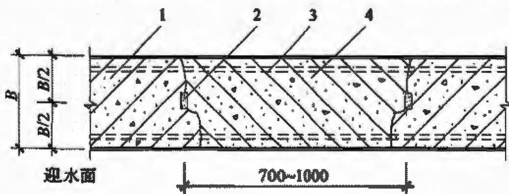
图 5.2.5-3 后浇带防水构造(三)
