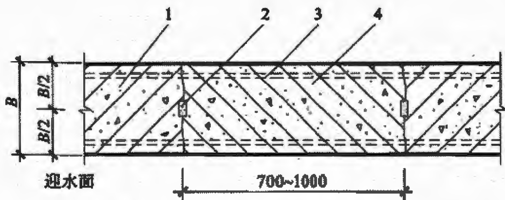
图 5.2.5-1 后浇带防水构造(一)
