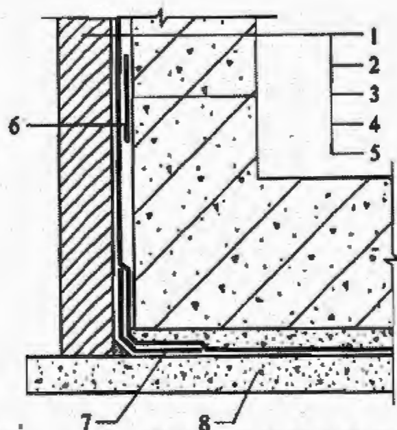
图 4.4.5-2 防水涂料外防内涂构造
