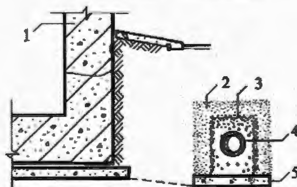
图 6.2.5-2 离墙盲沟设置
