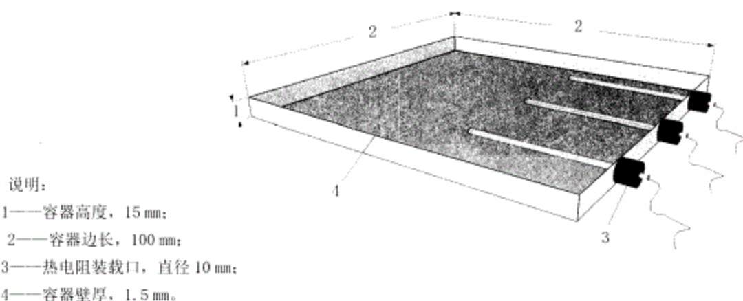
图 B.1 试验容器简图
