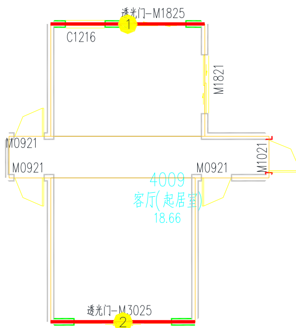
图 7.2-1 房间围护结构示意图
