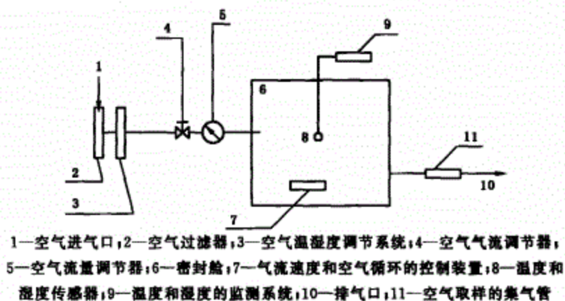
图 A.1 小型环境试验箱示意图
