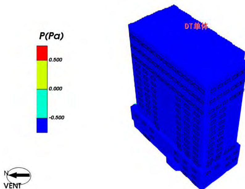
图 5.4-4 建筑背风面外窗表面风压云图-过渡季
