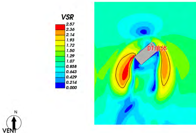
图 5.2-2 1.5 米高处风速放大系数云图
