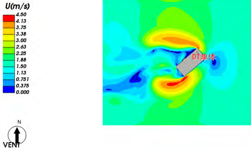
图 5.4-1 计算域内-1.5 米高度水平面风速云图-过渡季
