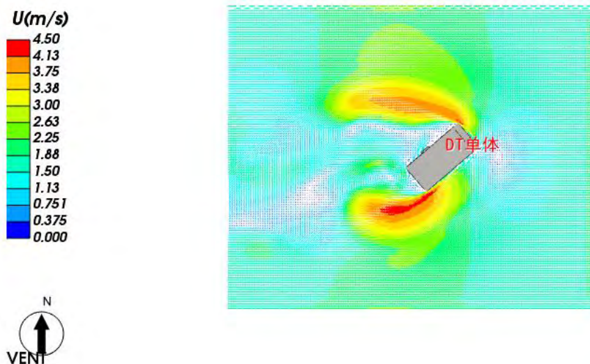
图 5.4-2 计算域内-1.5 米高度水平面风速矢量图
