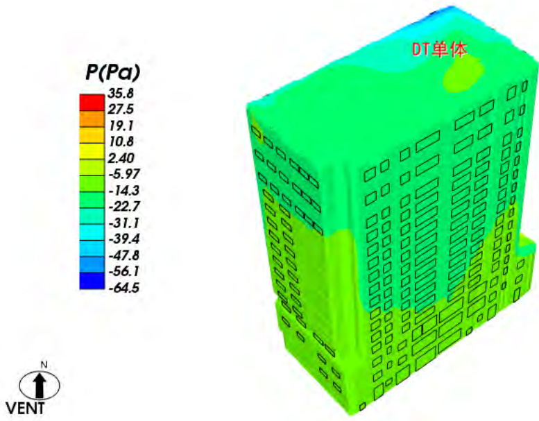
图 5.2-5 建筑背风面风压云图
