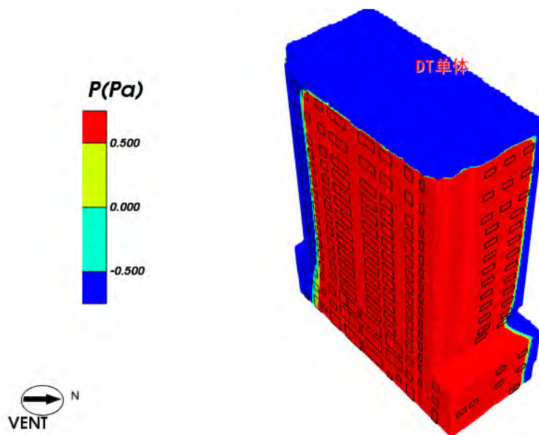
图 5.4-3 建筑迎风面外窗表面风压云图-过渡季
