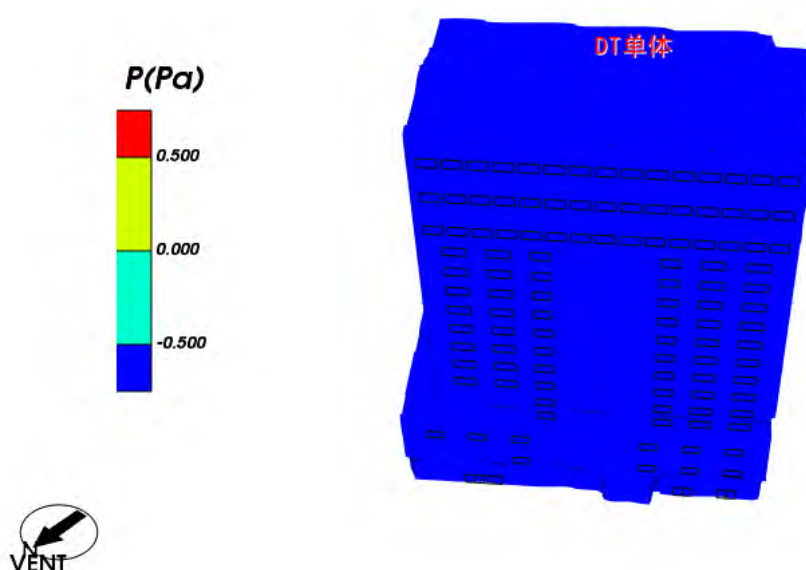
图 5.3-4 建筑背风面外窗表面风压云图-夏季
