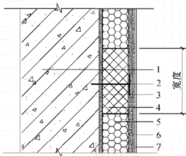
图 5.0.1 防火隔离带基本构造
