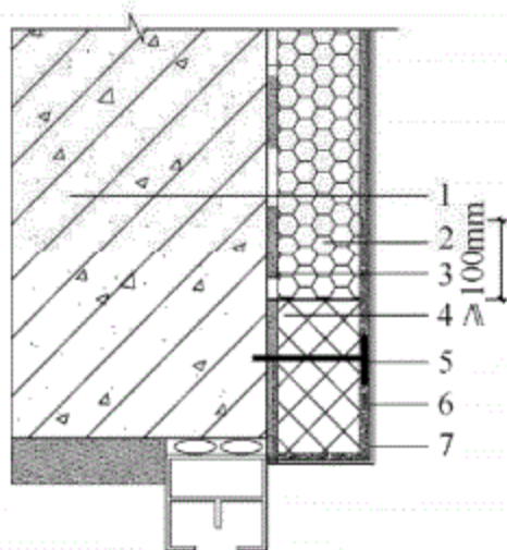
图 5.0.9 门窗洞口上部 防火隔离带做法（一）
