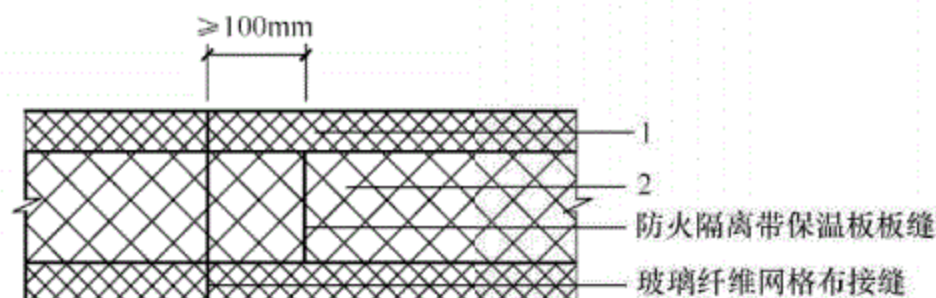
图 5.0.7-2 防火隔离带网格布水平方向对接
