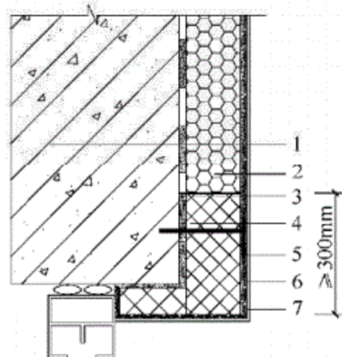
图 5.0.10 门窗洞口上部防火 隔离带做法（二）
