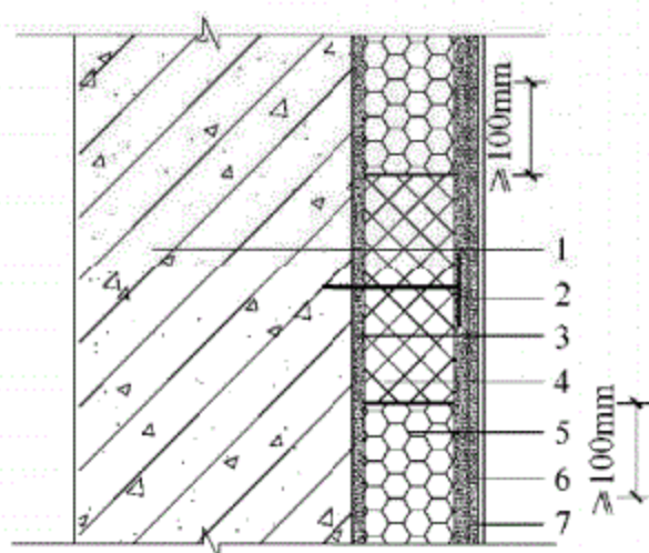
图 5.0.7-1 防火隔离带网格布垂直方向搭接
