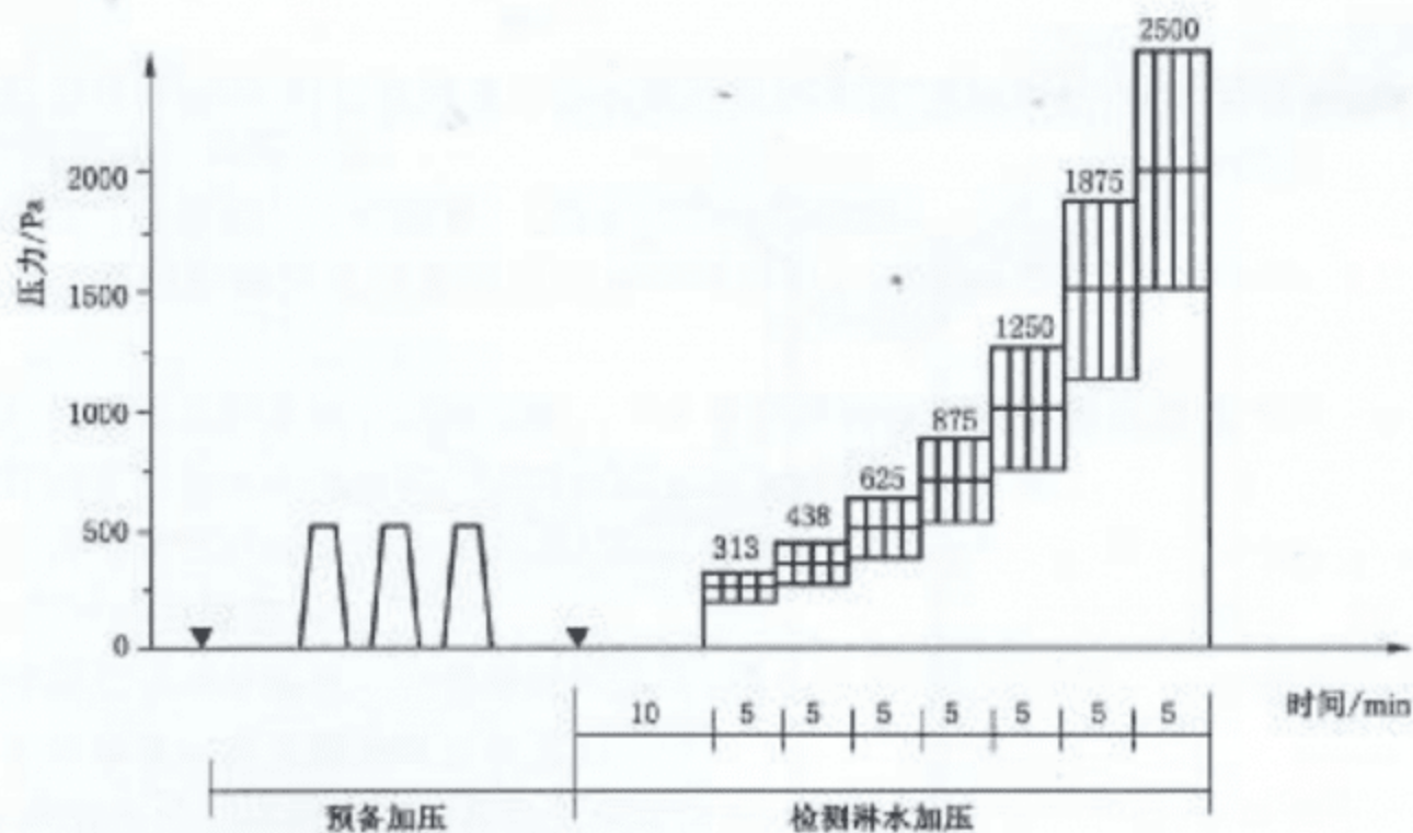
图 5 波动加压示意图
