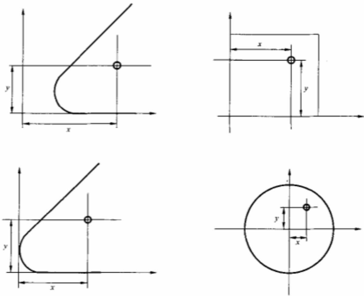
图 4 圆心位置表示方法
