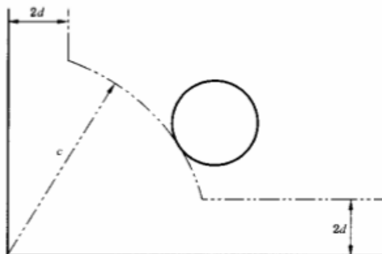
图 3 孔的边部距玻璃角部的距离示意图
