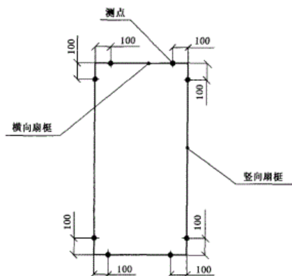
图 1 门窗扇与框的相对位置测点示意
