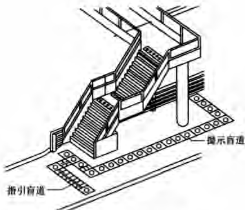
图 4-1 人行天桥提示盲道示意图
