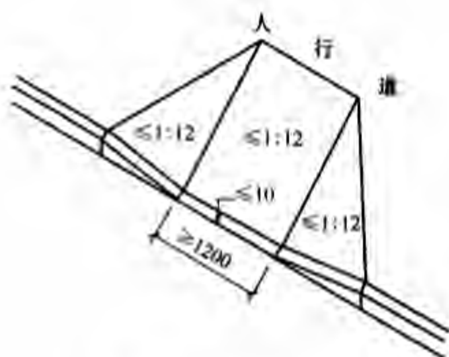
图 3-2 三面坡缘石坡道
