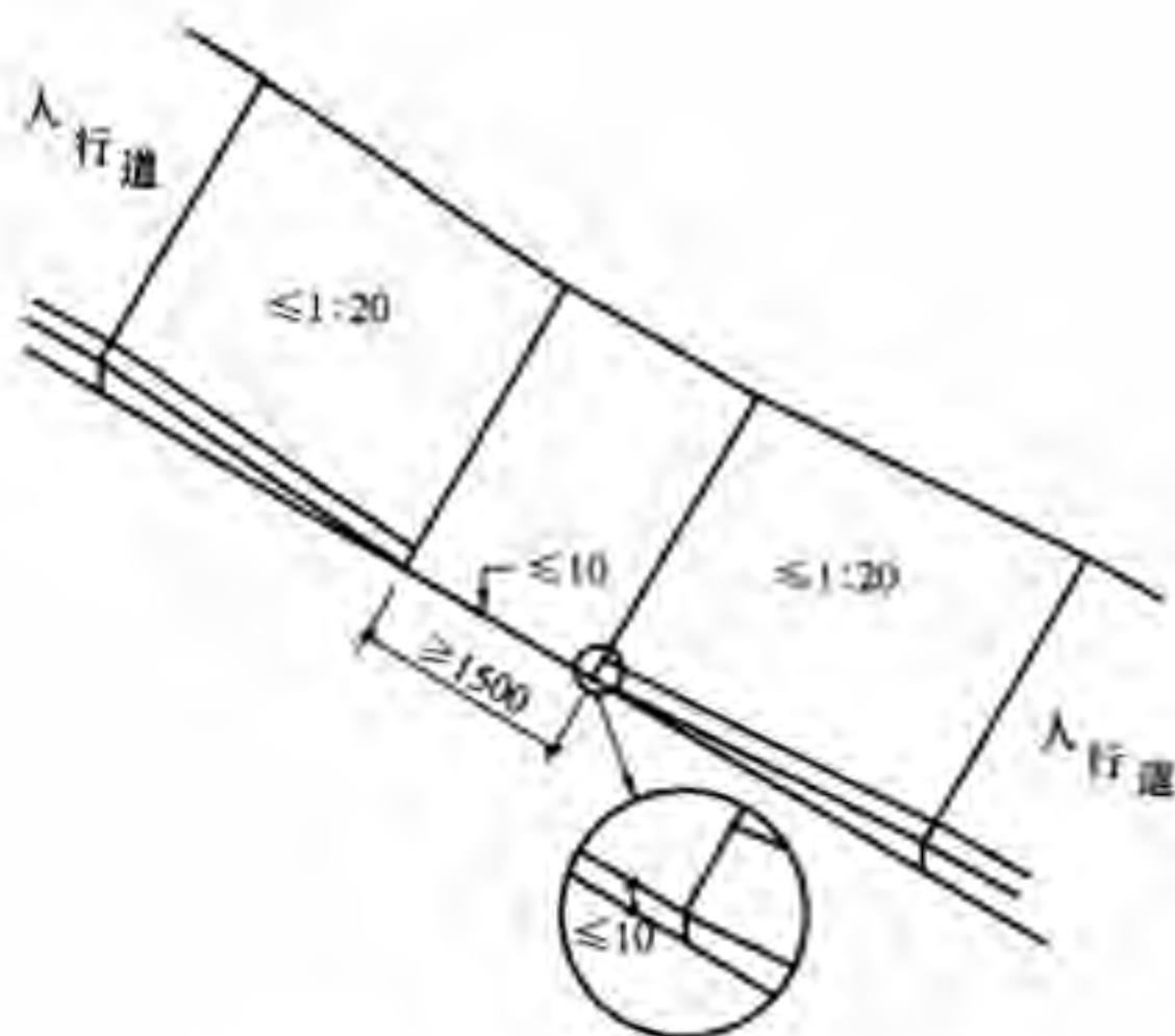
图 3-1 全宽式单面坡缘石坡道
