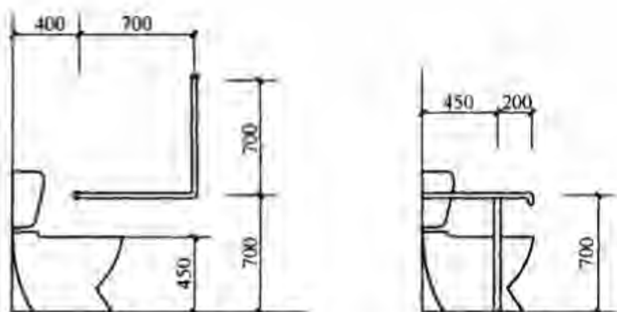
图 3-5 坐式便器及安全抓杆
