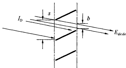
图 C. 10.2 百叶系统透空部分的直射辐射示意
