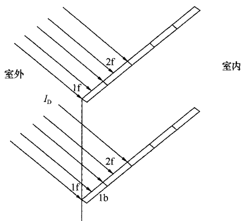
图 8 百叶板条受到直射辐射的部分
