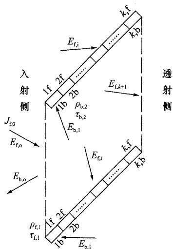
图7 模型单元中百叶板条的分割示意
