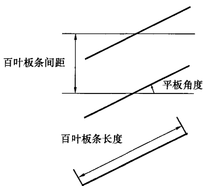
图 6 百叶系统中的板条几何形状和位置
