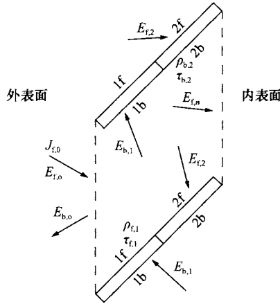
图9 用于计算机算法的百叶遮阳板示意
