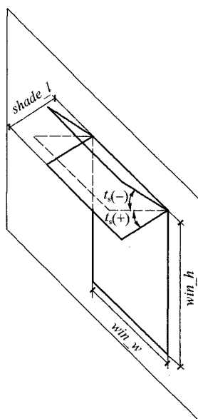
图 C. 8. 1 水平遮阳板计算参数示意
