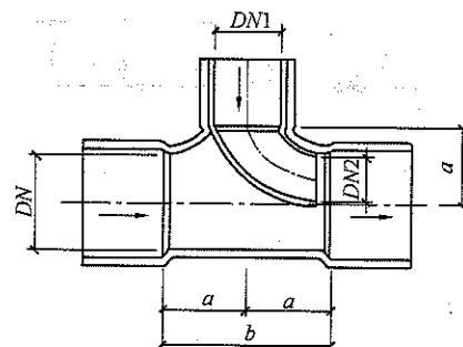
图 3 导流三通
