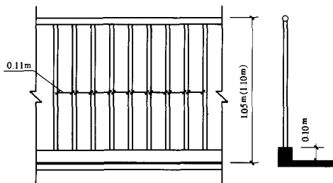
图 6.6.3-2 垂直栏杆
