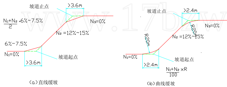
图 4.1.8 缓坡
