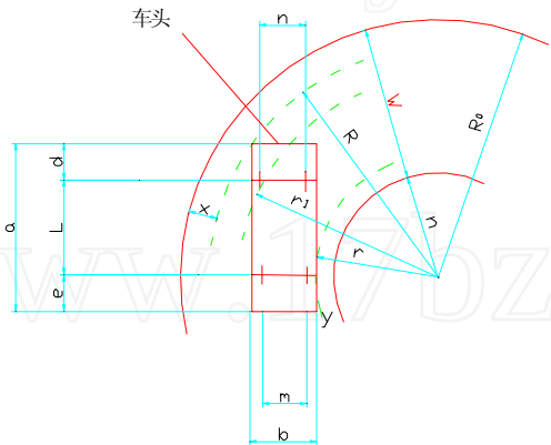
图 4.1.10 汽车环道平面
