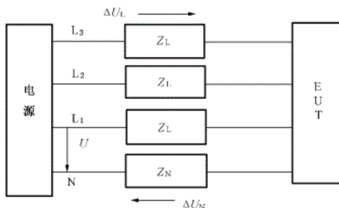
图 1 单相设备谐波电流发射测量电路
