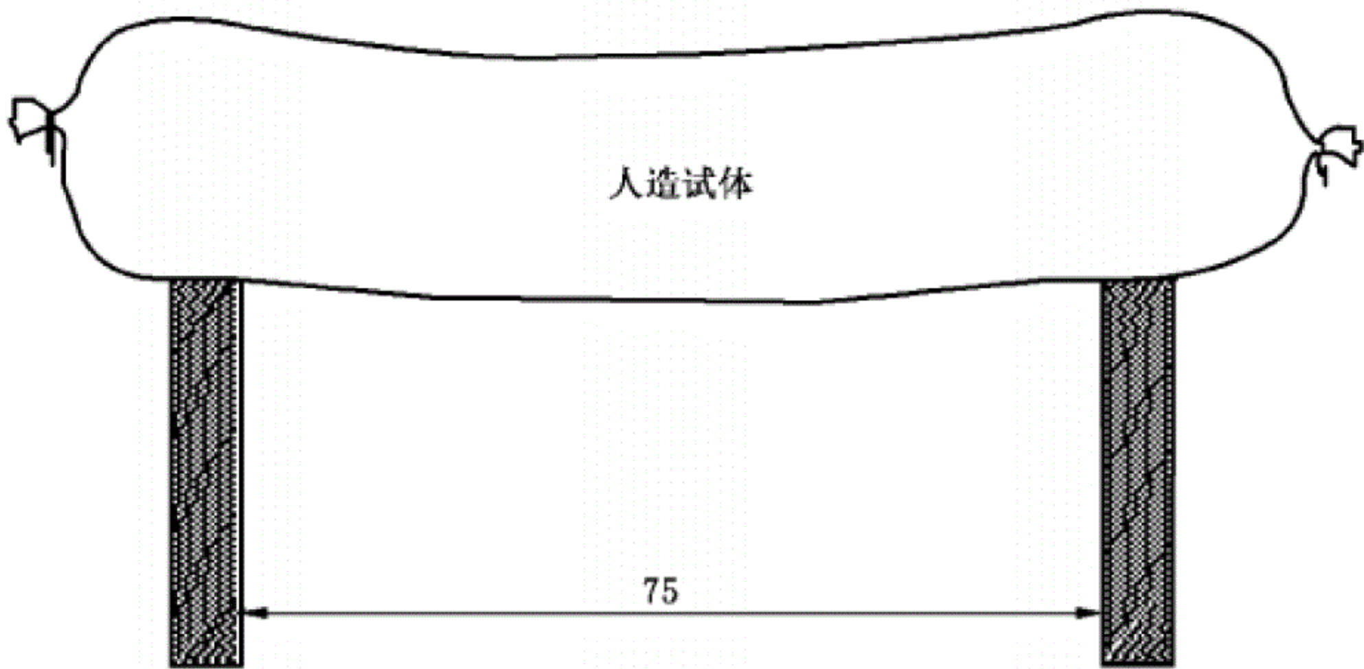
图 A.1 人造试体柔曲性试验示意图
