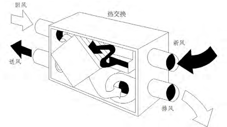
图 13 新风热回收装置示意图
