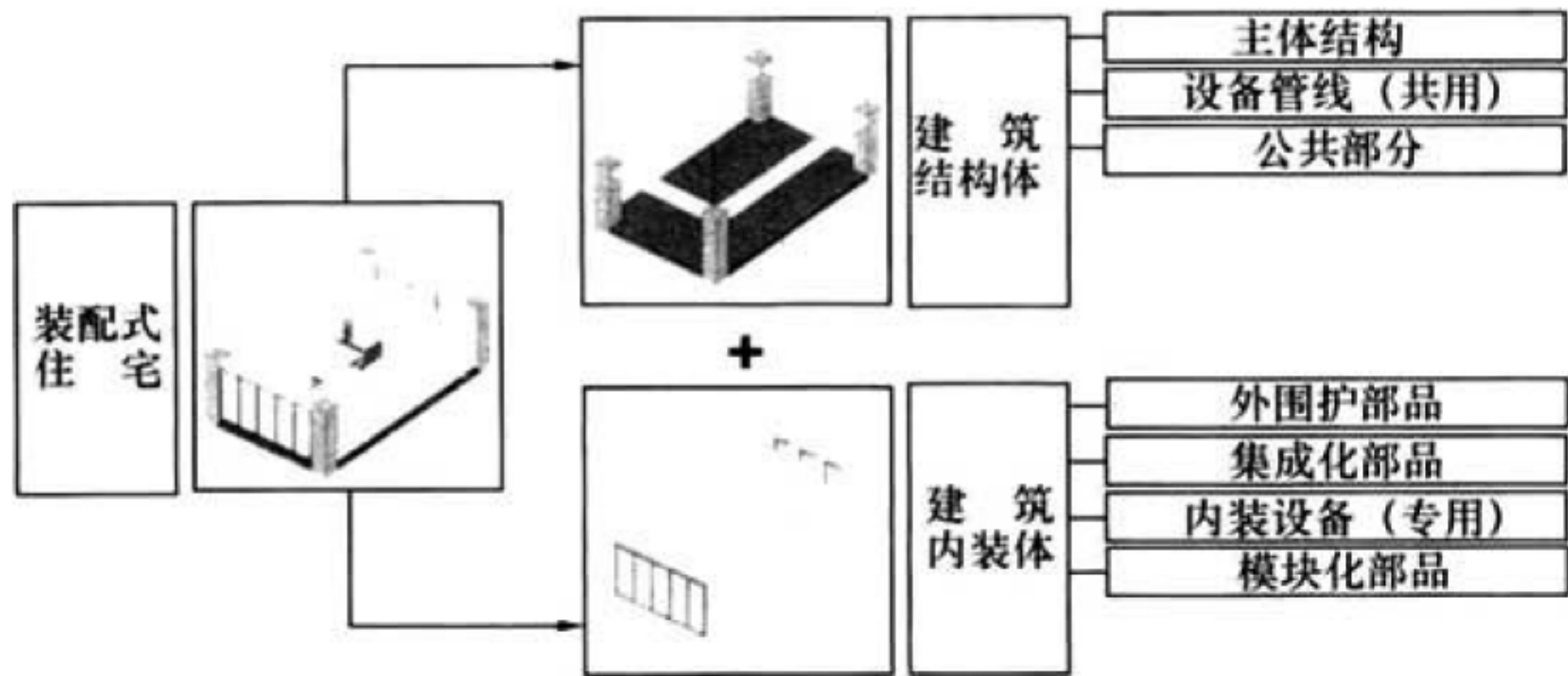
图1 框架结构建筑体系与建筑内装体的建筑体系构成示意
