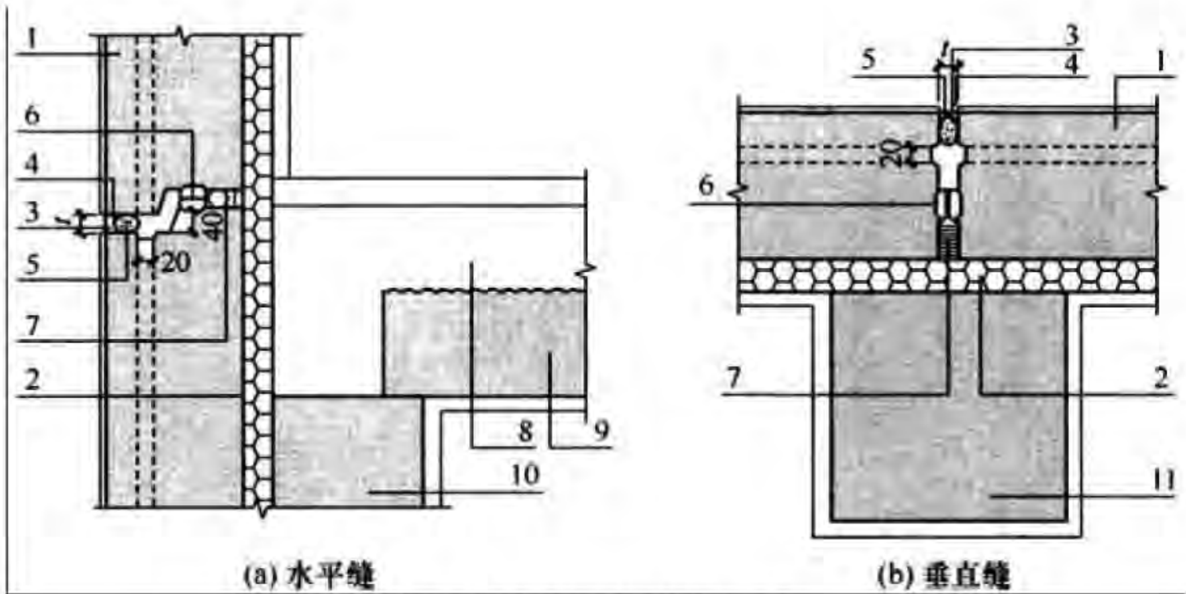
图3 预制外挂墙板板缝构造示意
