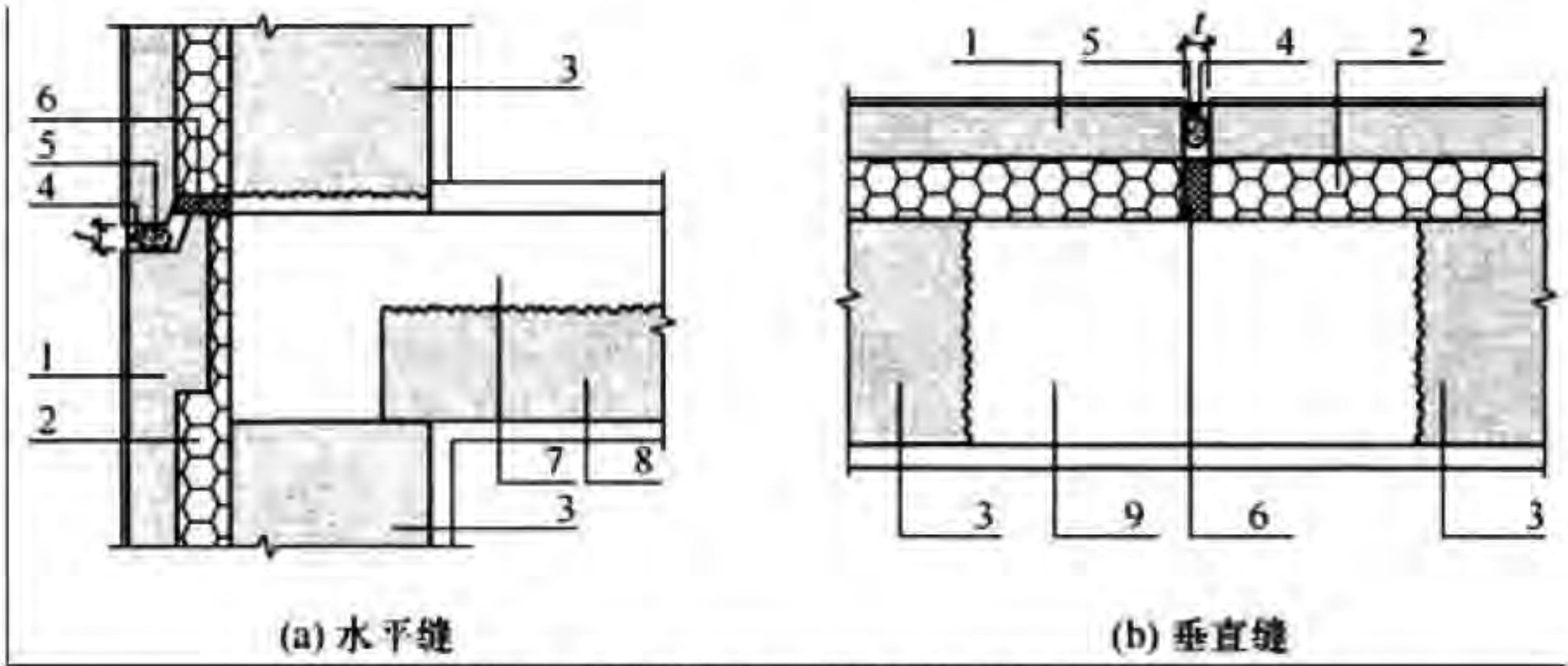
图2 预制承重夹心外墙板板缝构造示意
