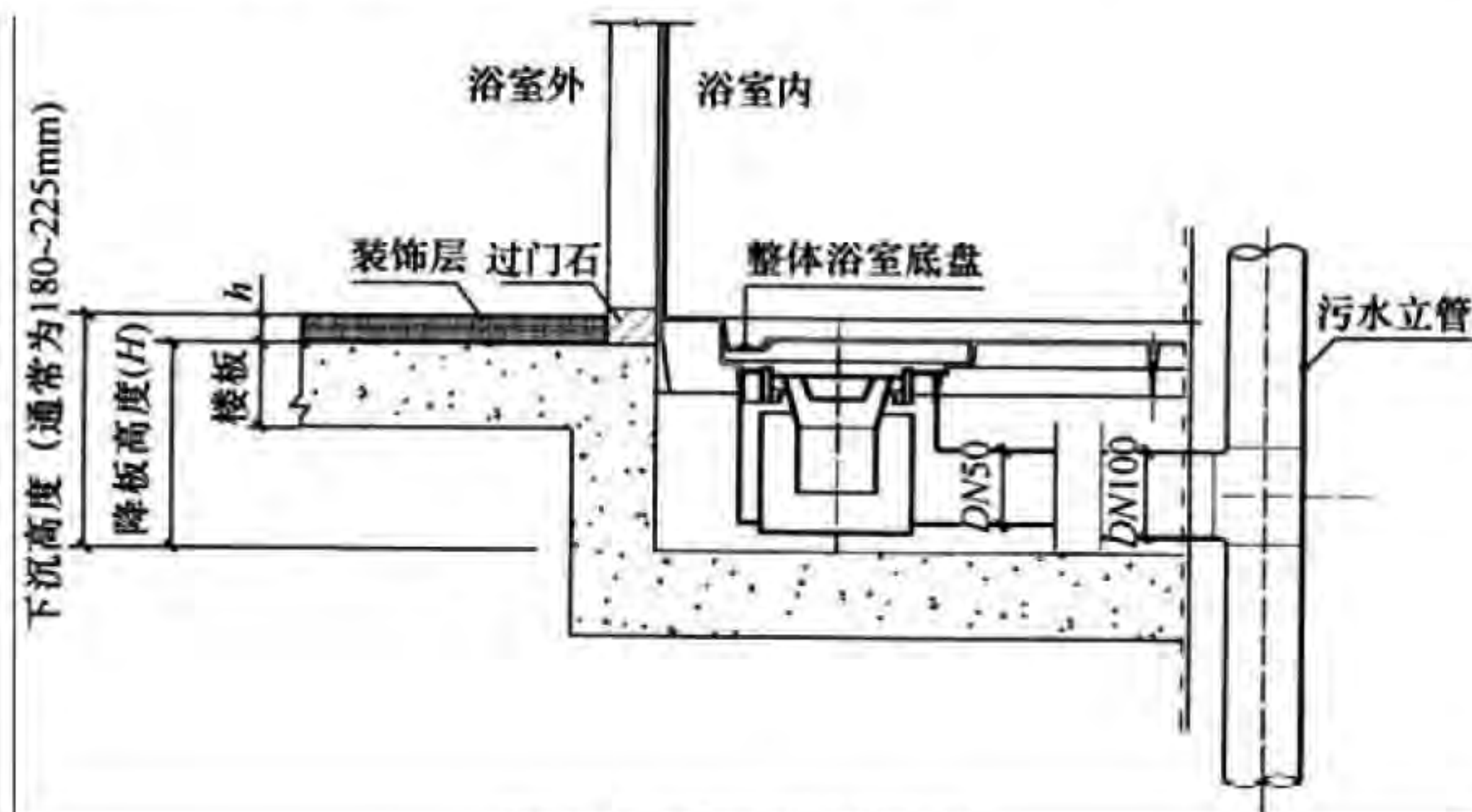
图4 整体浴室同层排水构造示意
