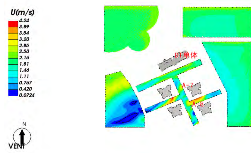
图 5.3-1 人行区域-1.5 米高度水平面风速云图-夏季
