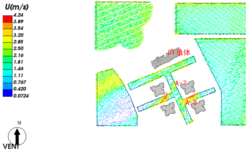
图 5.3-3 人行区域-1.5 米高度水平面风速矢量图
