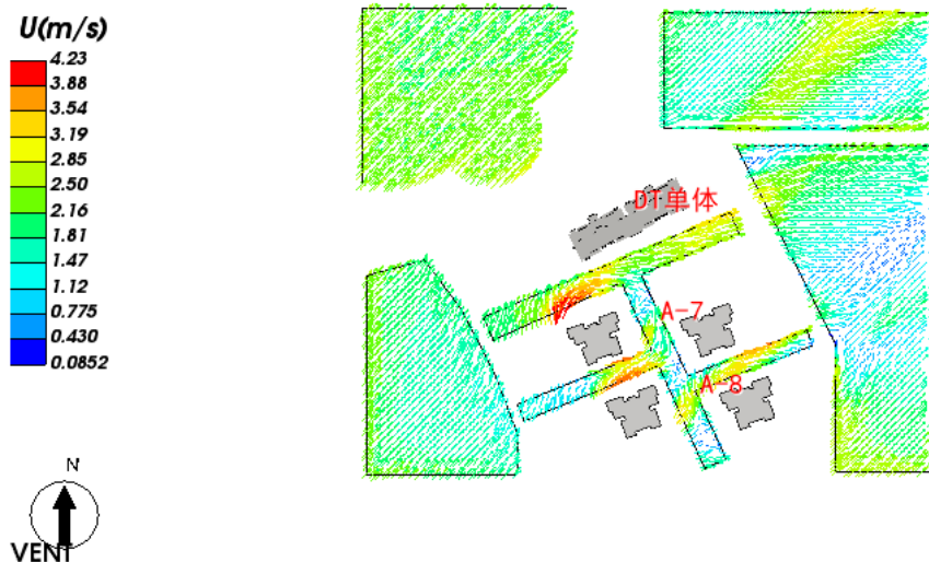
图 5.4-3 人行区域-1.5 米高度水平面风速矢量图
