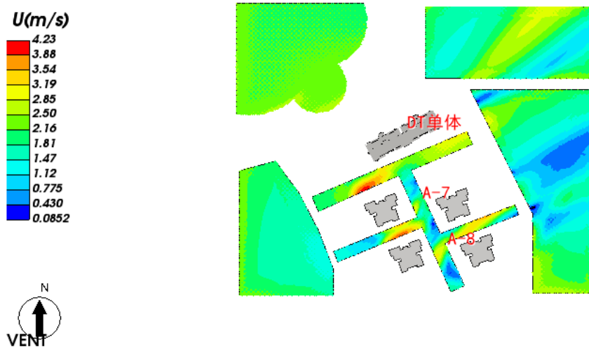
图 5.4-1 人行区域-1.5 米高度水平面风速云图-过渡季
