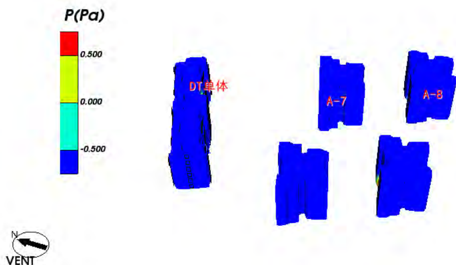
图 5.3-6 建筑背风面外窗表面风压云图-夏季
