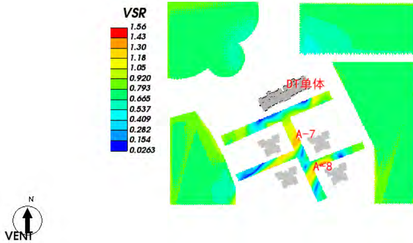
图 5.2-3 人行区域-1.5 米高度水平面风速放大系数云图-冬季
