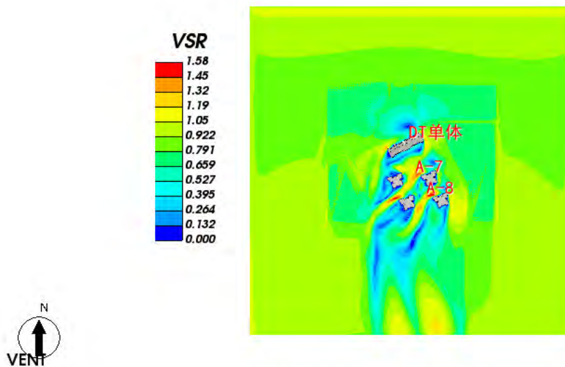
图 5.2-4 1.5 米高处风速放大系数云图
