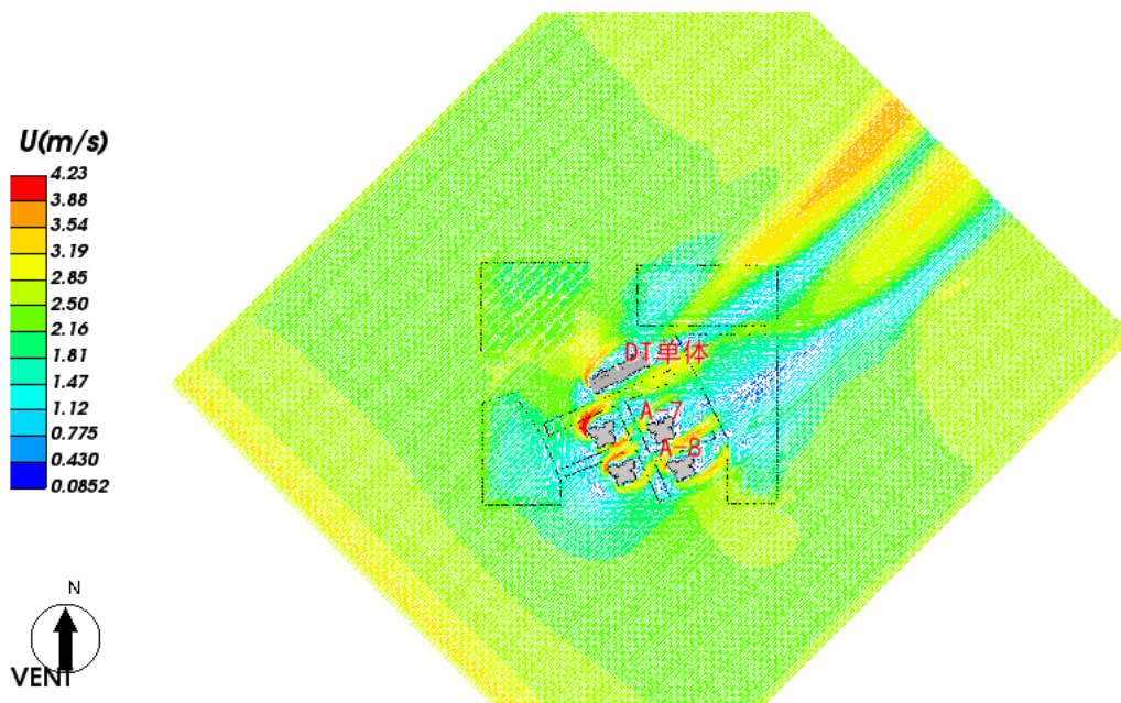
图 5.4-4 计算域内-1.5 米高度水平面风速矢量图
