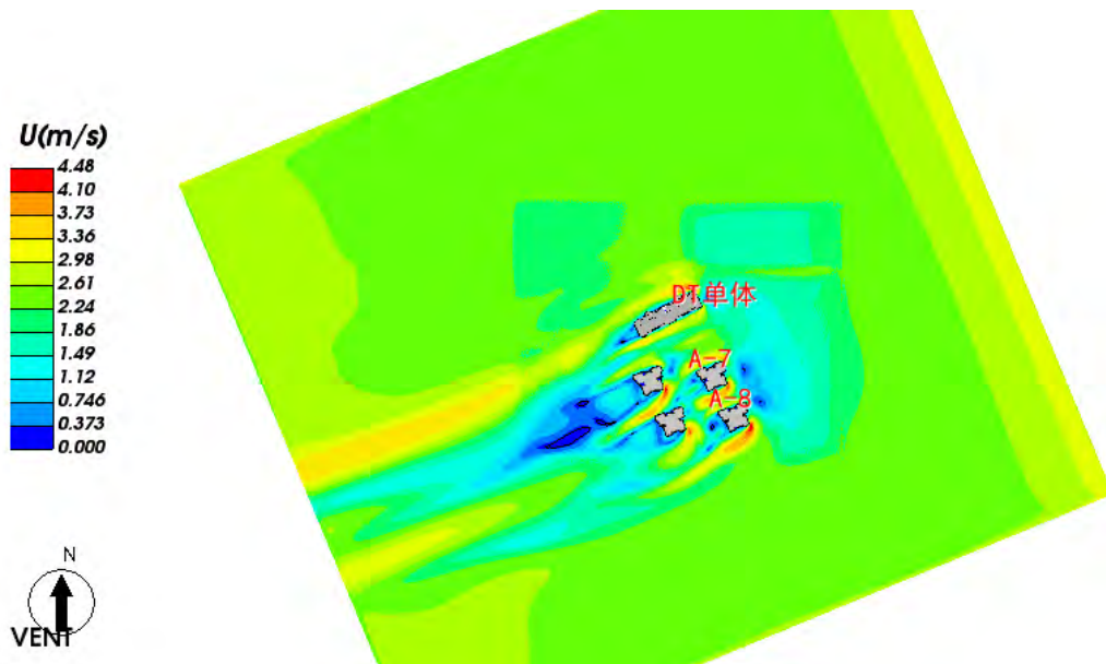
图 5.3-2 计算域内-1.5 米高度水平面风速云图-夏季
