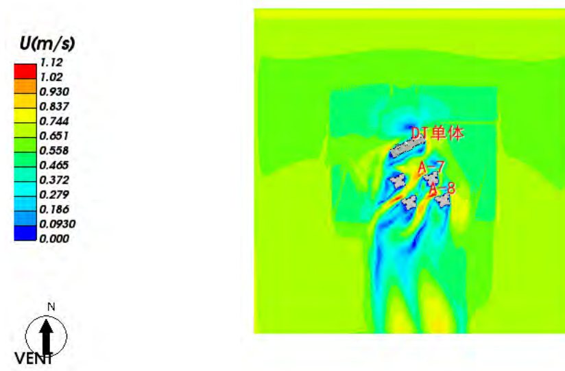
图 5.2-2 计算域内-1.5 米高度水平面风速云图-冬季
