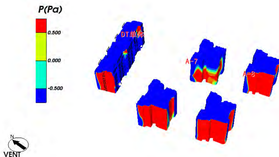
图 5.4-5 建筑迎风面外窗表面风压云图-过渡季
