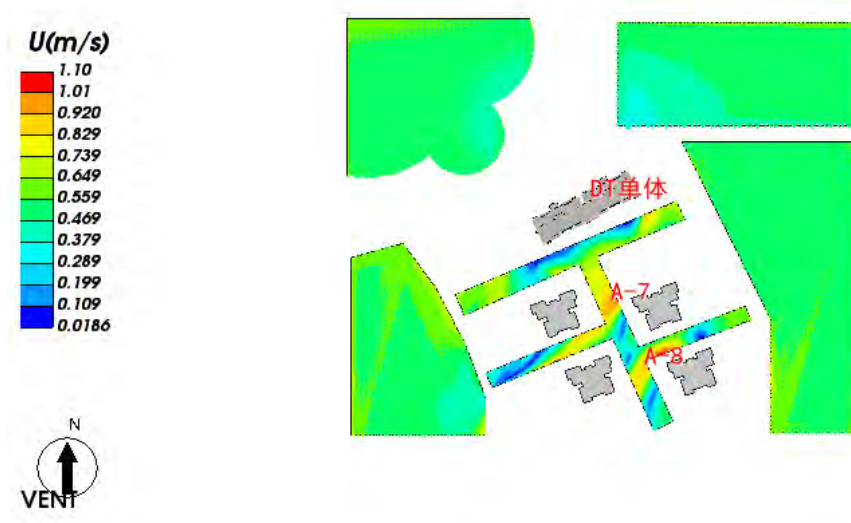
图 5.2-1 人行区域-1.5 米高度水平面风速云图-冬季
