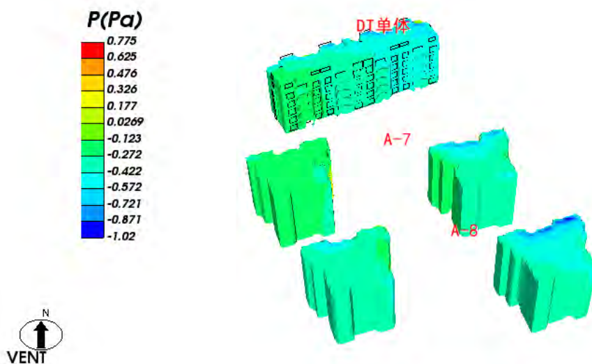
图 5.2-7 建筑背风面风压云图
