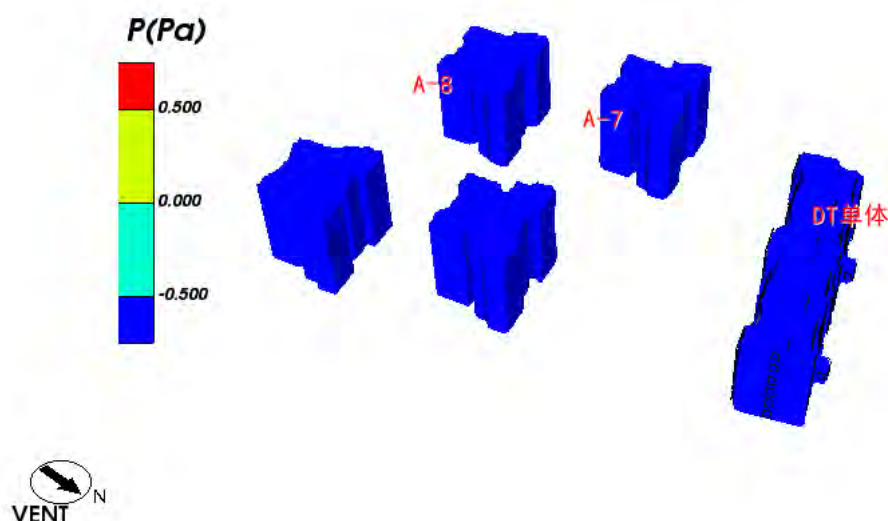
图 5.4-6 建筑背风面外窗表面风压云图-过渡季
