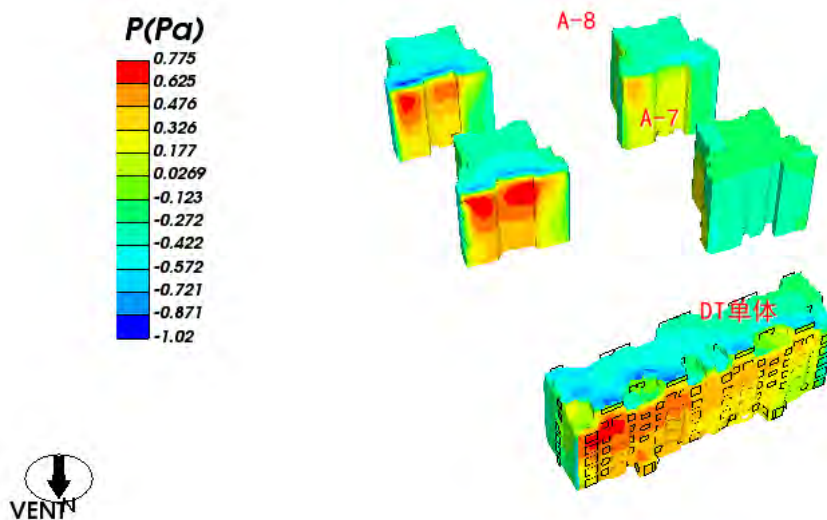
图 5.2-6 建筑迎风面风压云图
