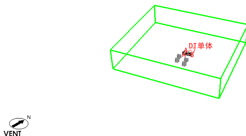
图 4.1-2 夏季工况风场计算域图示
