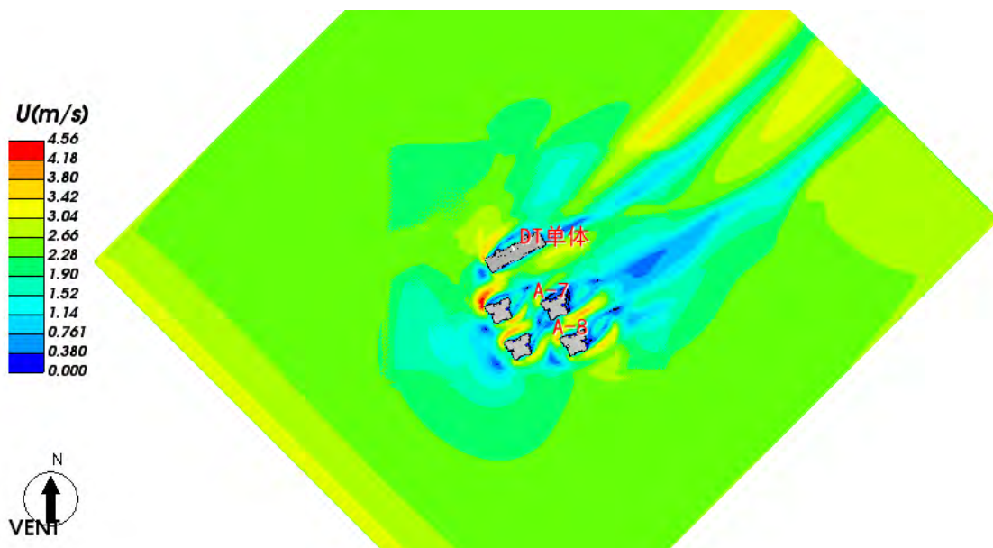
图 5.4-2 计算域内-1.5 米高度水平面风速云图-过渡季
