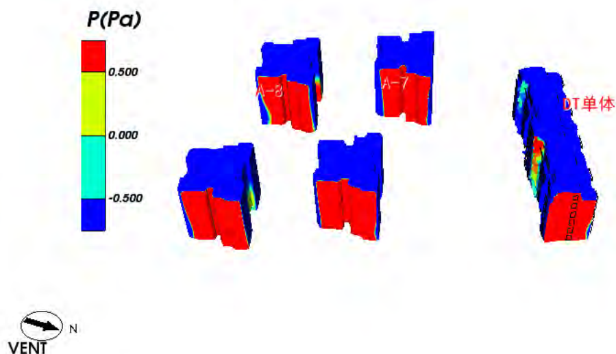
图 5.3-5 建筑迎风面外窗表面风压云图-夏季
