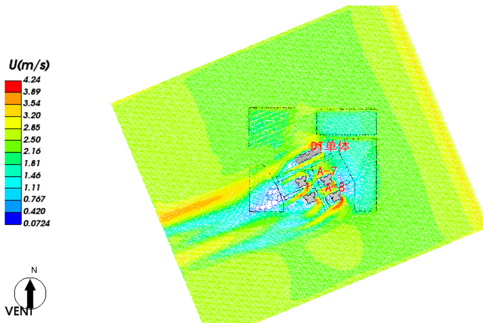
图 5.3-4 计算域内-1.5 米高度水平面风速矢量图
