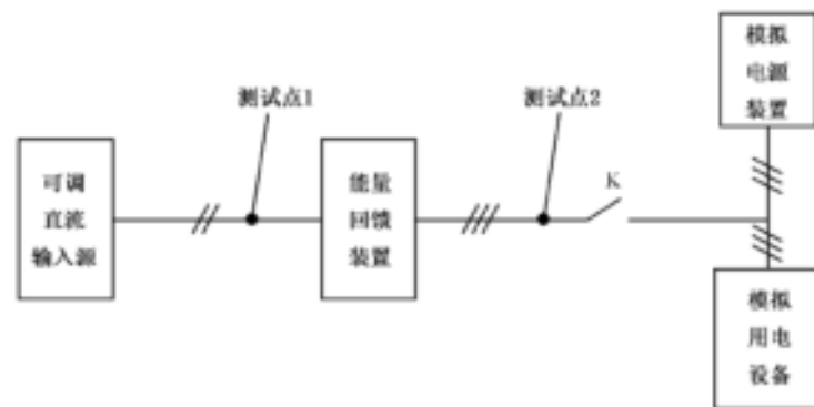
图 1 性能指标试验平台
