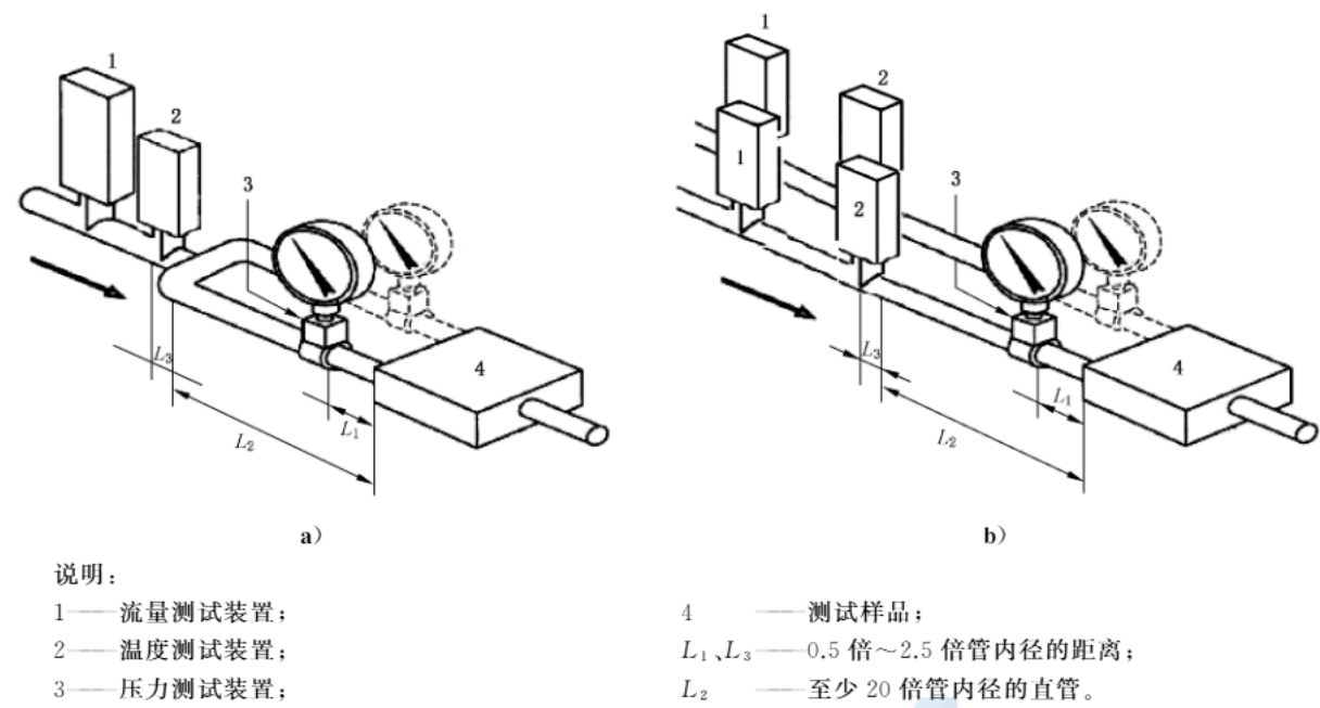
图 A.1 水嘴试验装置示意图
