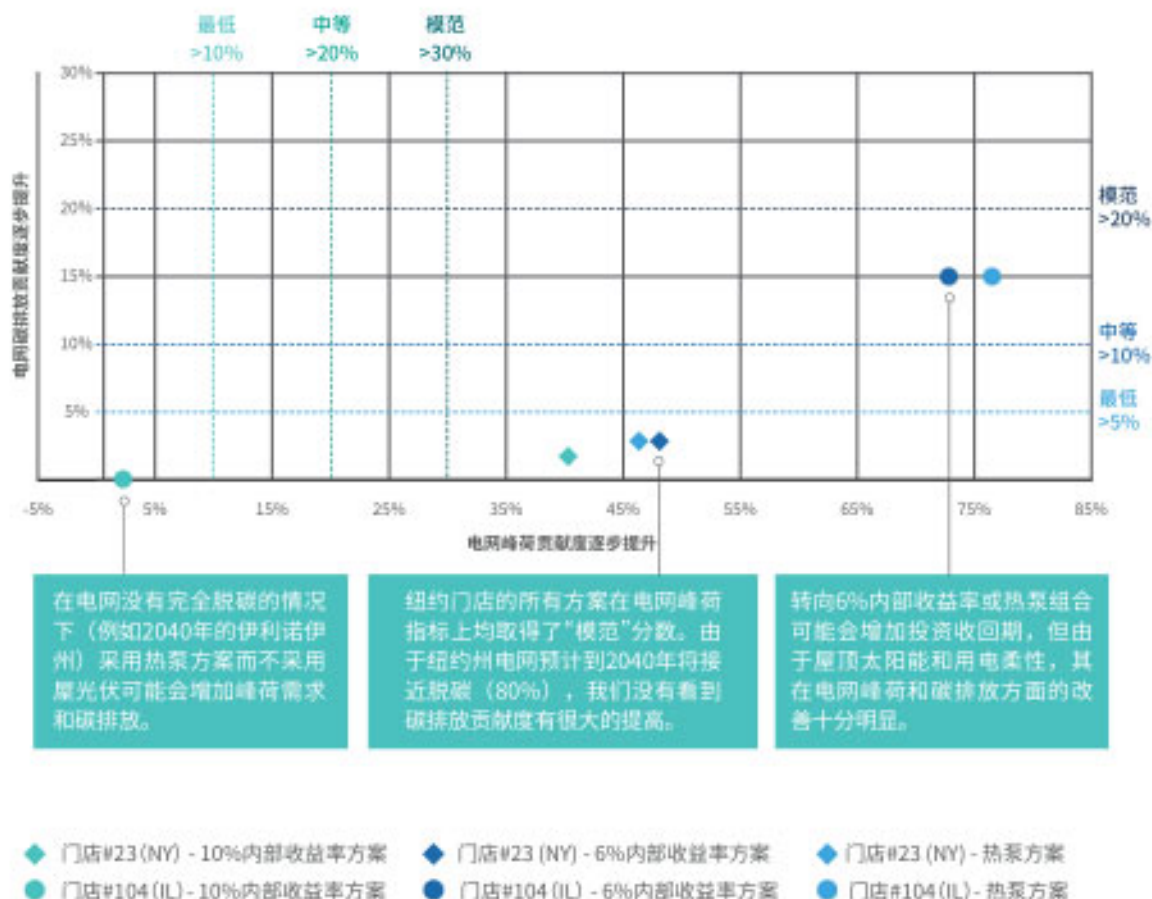
图23 不同方案的GridOptimal分数 门店#23（纽约）与门店#104（伊利诺斯州）
