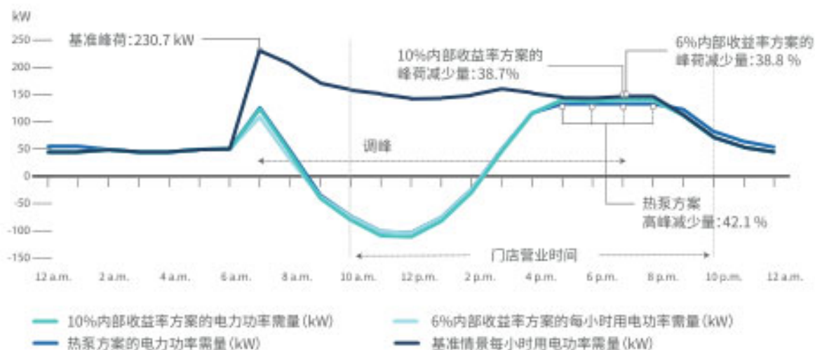
图20 门店#65(阿拉巴马州): 电力负荷对比 2019年12月12日 (冬日)
