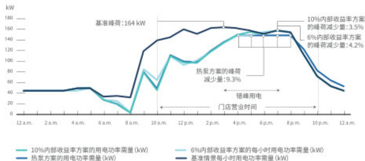
图21 门店#65(阿拉巴马州): 电力负荷对比 2019年10月1日 (温和日)
