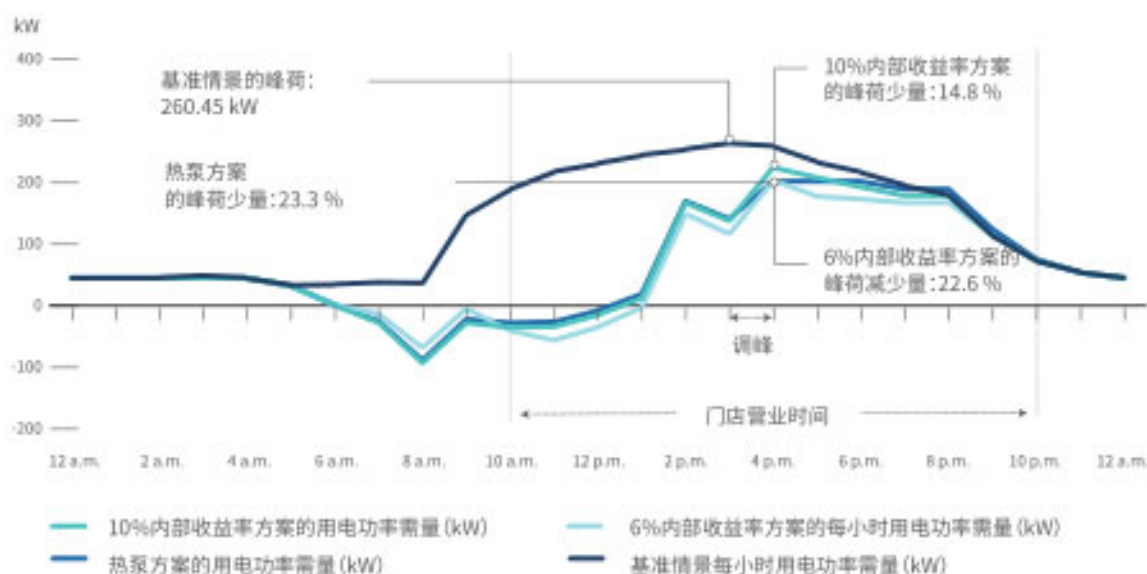
图19 门店#65(阿拉巴马州)：电力负荷对比
