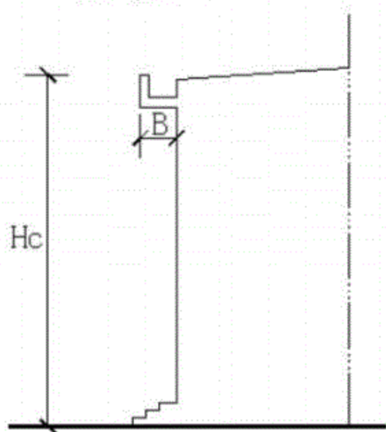
图一 挑檐屋面
