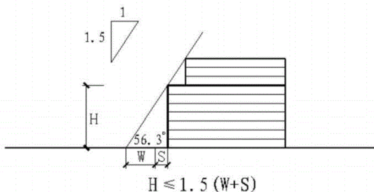
图五 沿路一般建筑高度的控制
