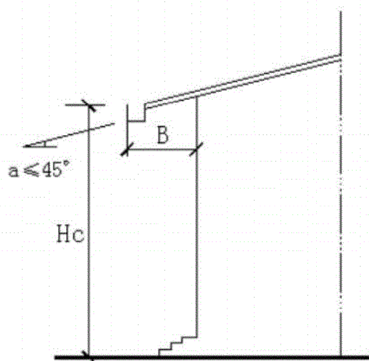
图三 屋面坡度小于 45^\circ (含 45^\circ )
