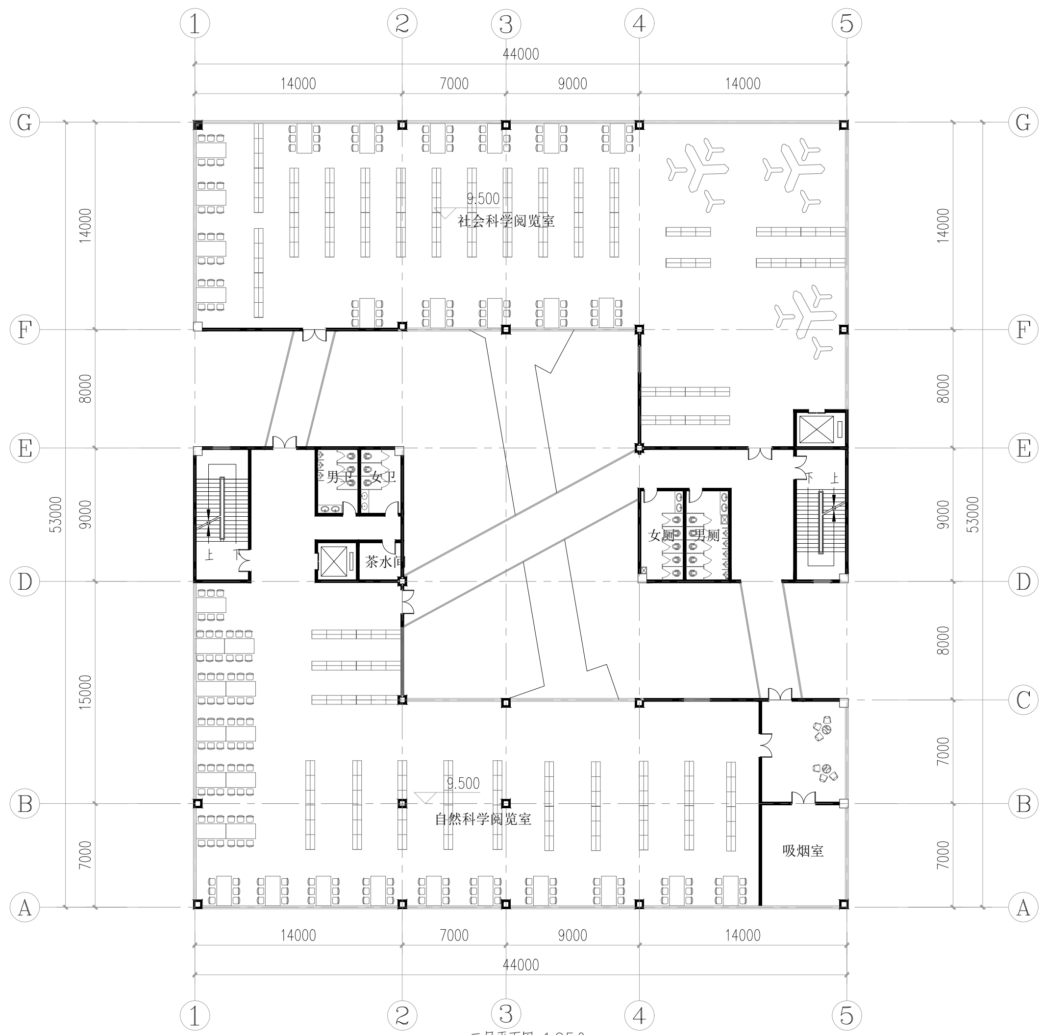
三层平面图 1:250
