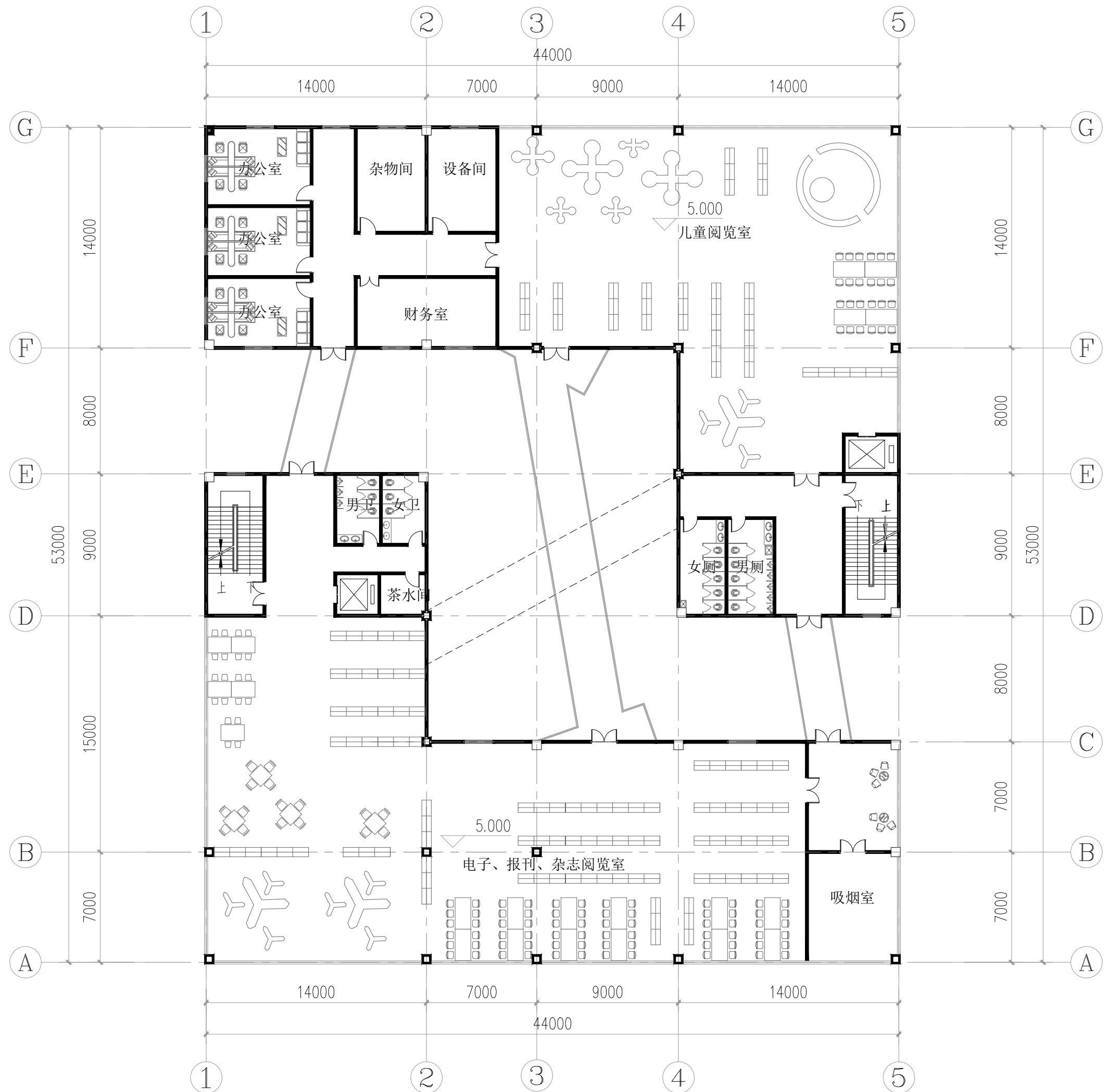
二层平面图 1:250
