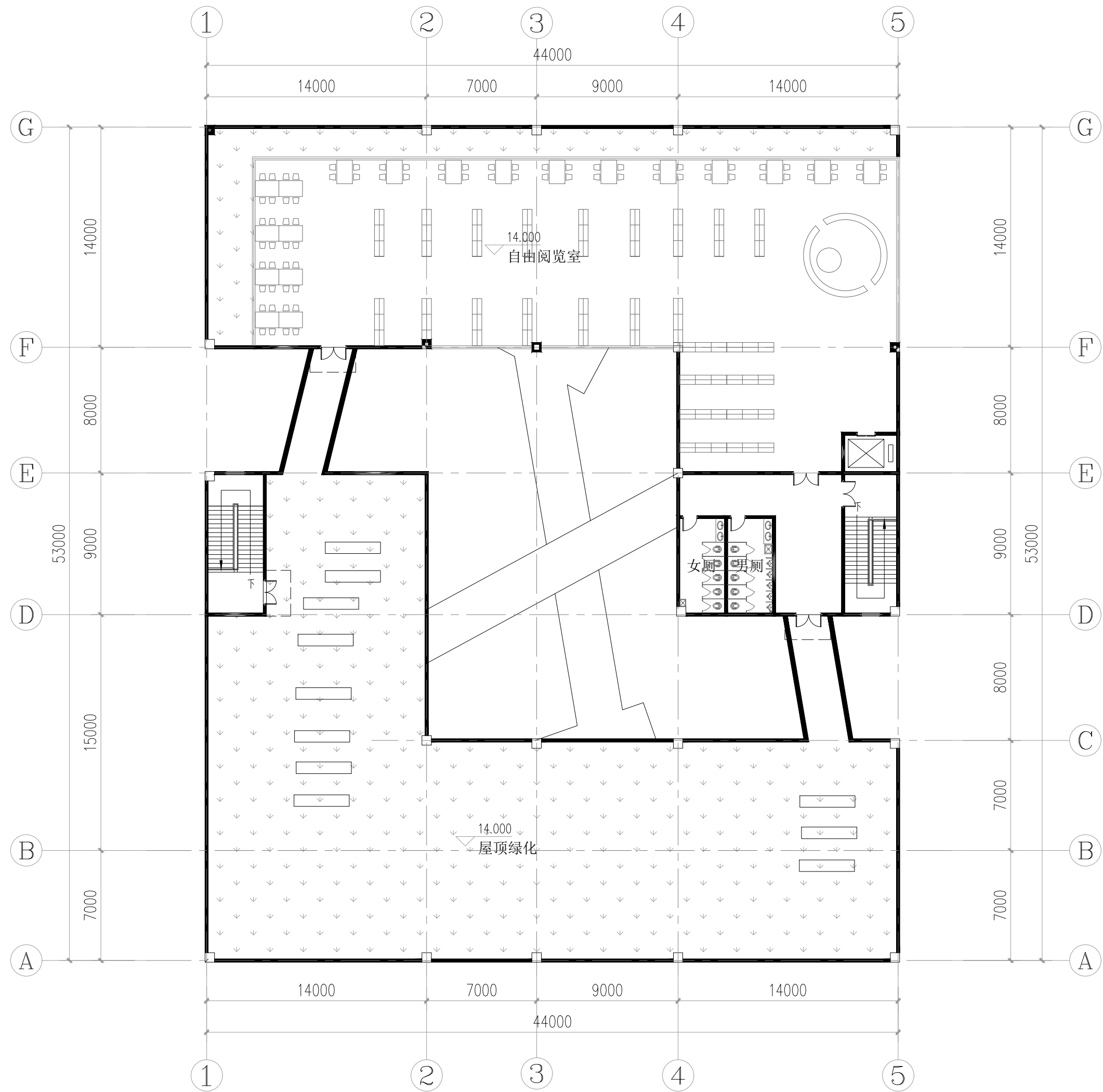
四层平面图 1:250
