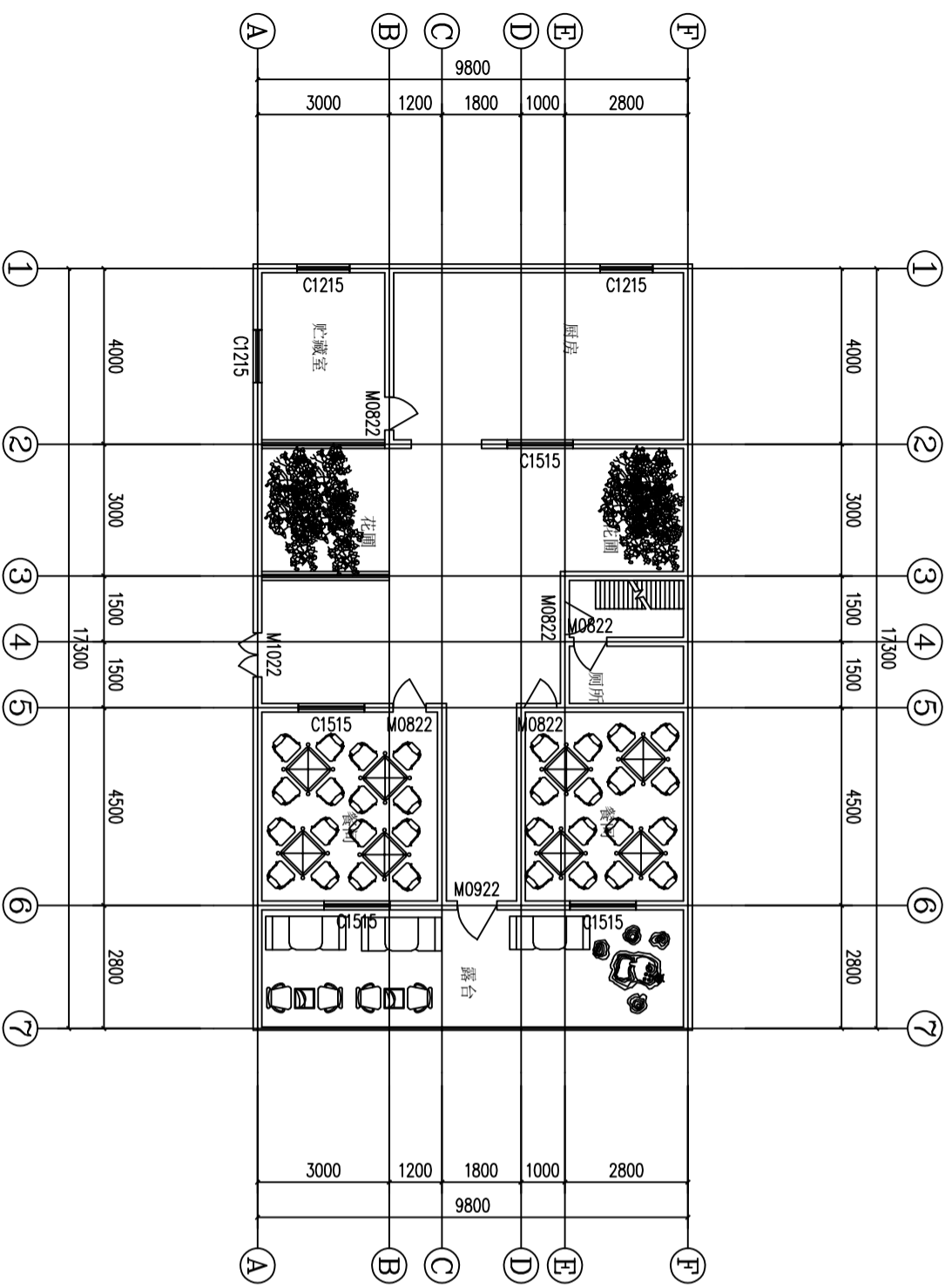
改造后的一层平面图
