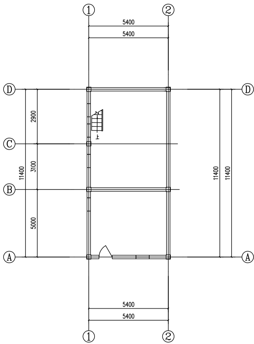
首层平面图 1: 100
