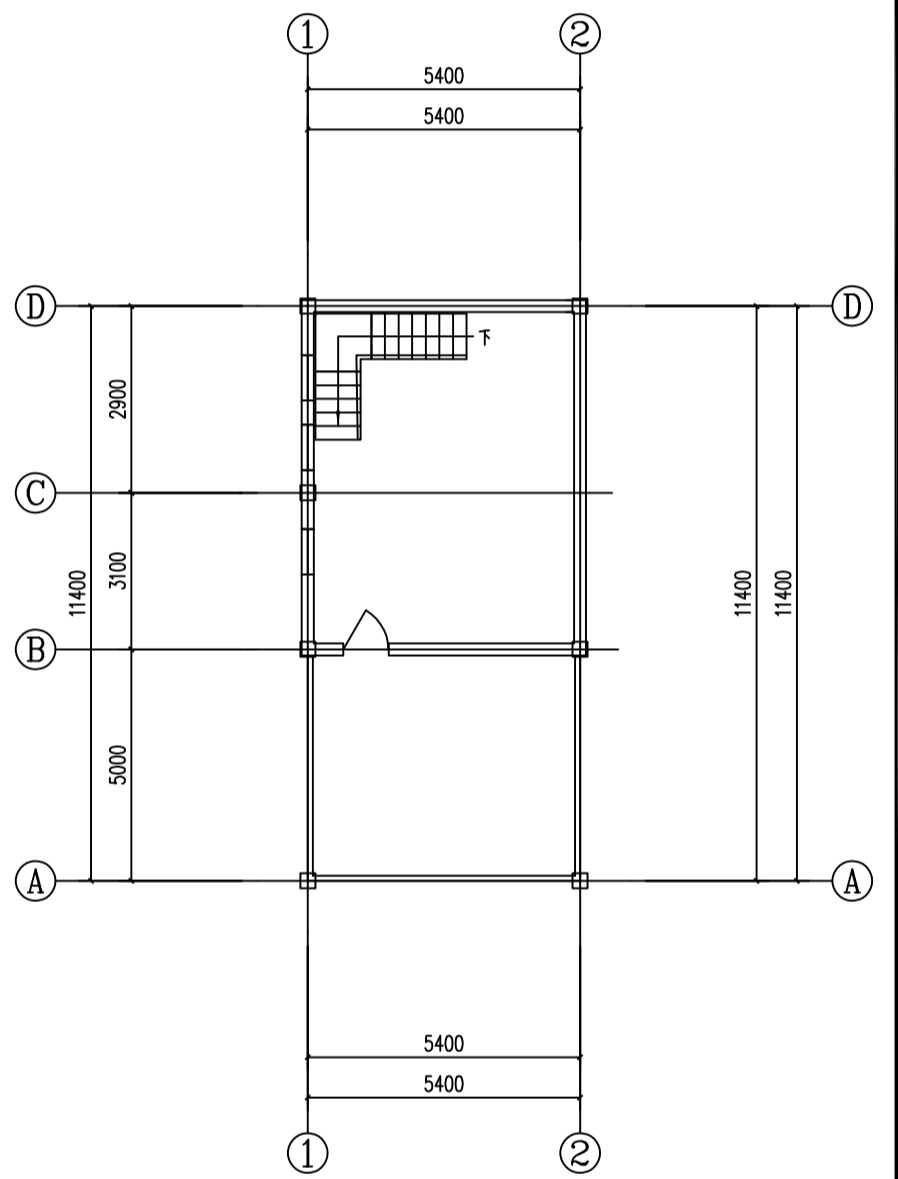
二层平面图 1: 100
