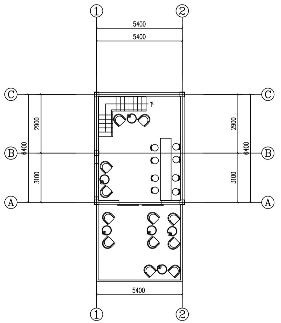
二层平面图 1: 100
