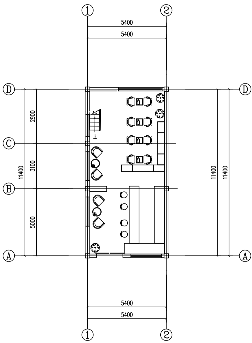
首层平面图 1: 100
