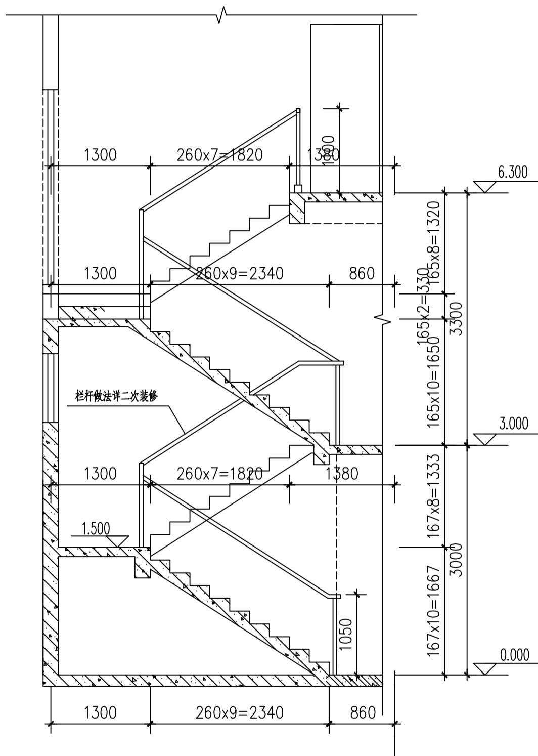
1-1剖面图 1:50
