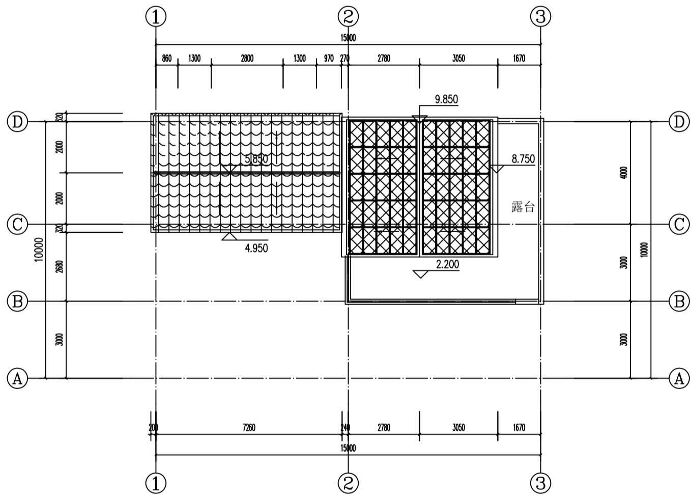
屋顶平面图
