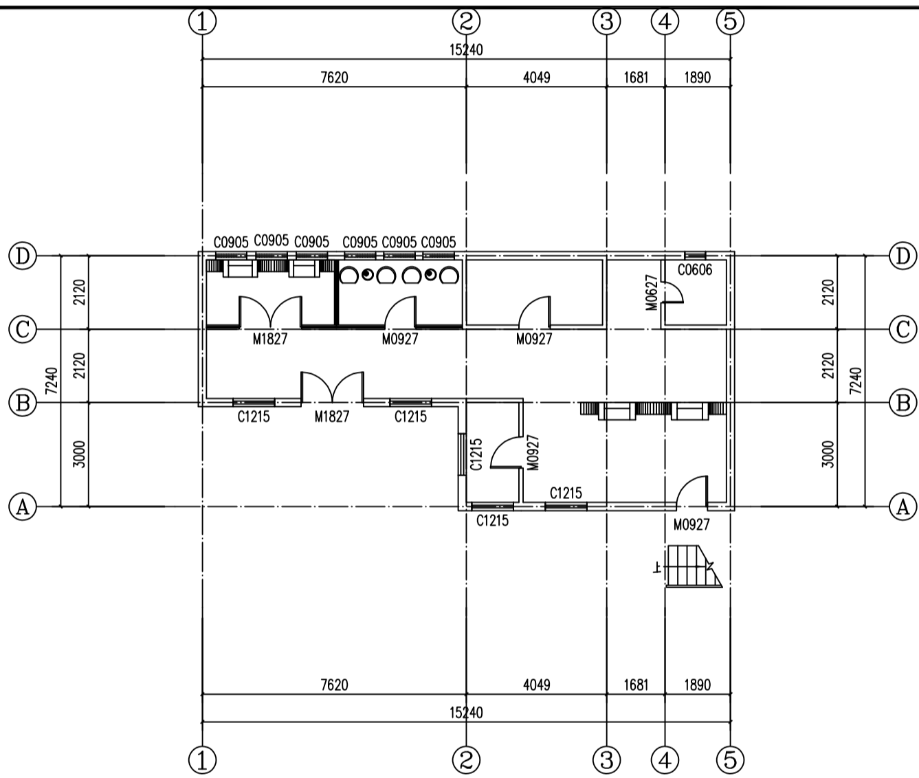
一层平面图 1:100
