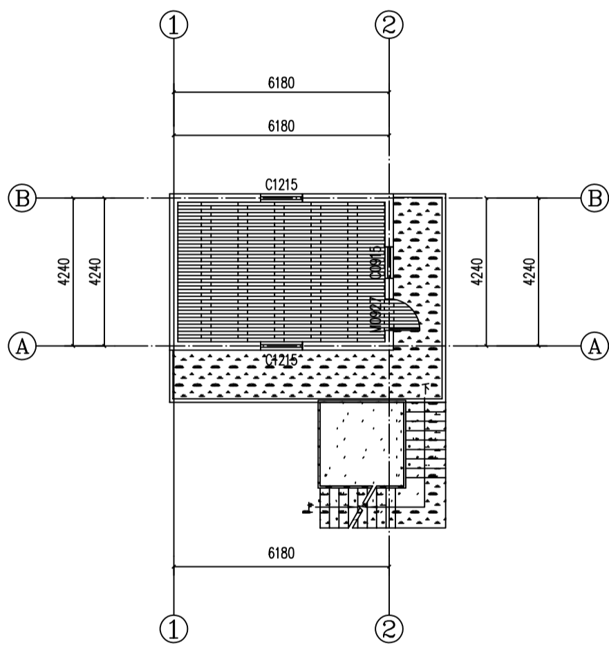
二层平面图 1:100
