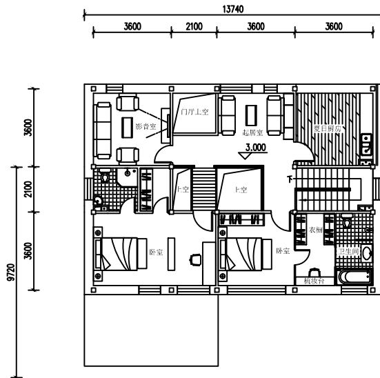
二层平面图 1:100
