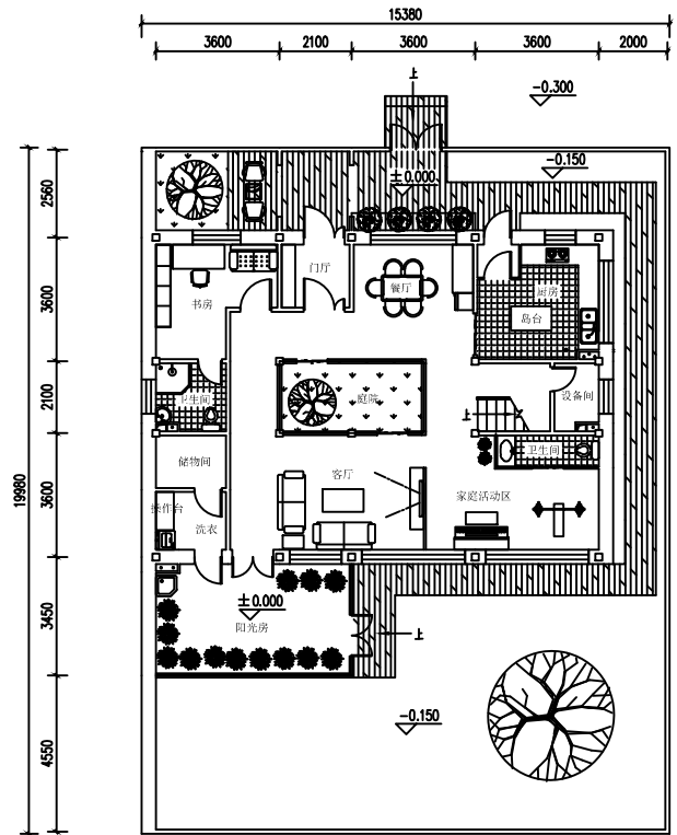
底层平面图 1:100
