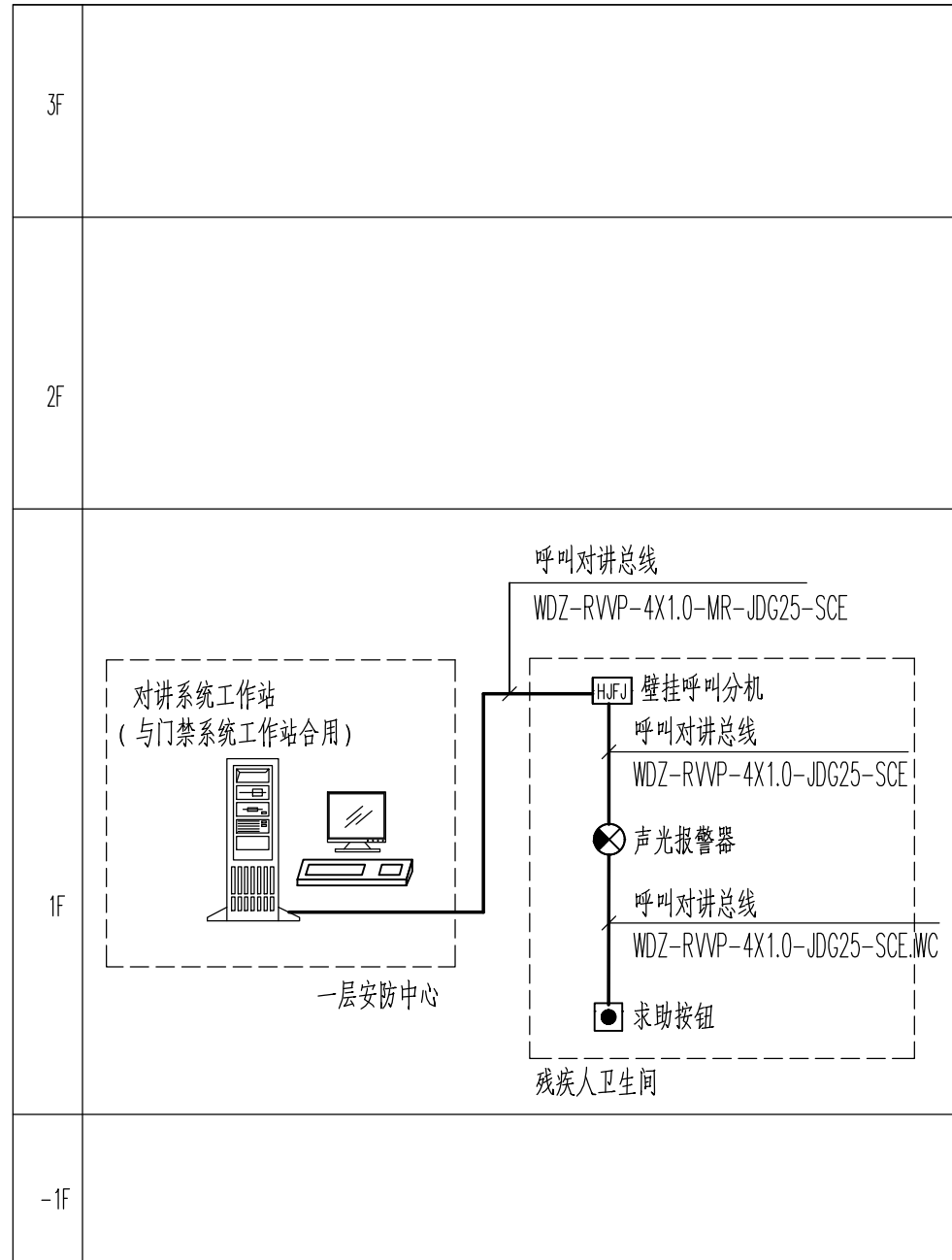
残疾人卫生间呼叫对讲系统图
