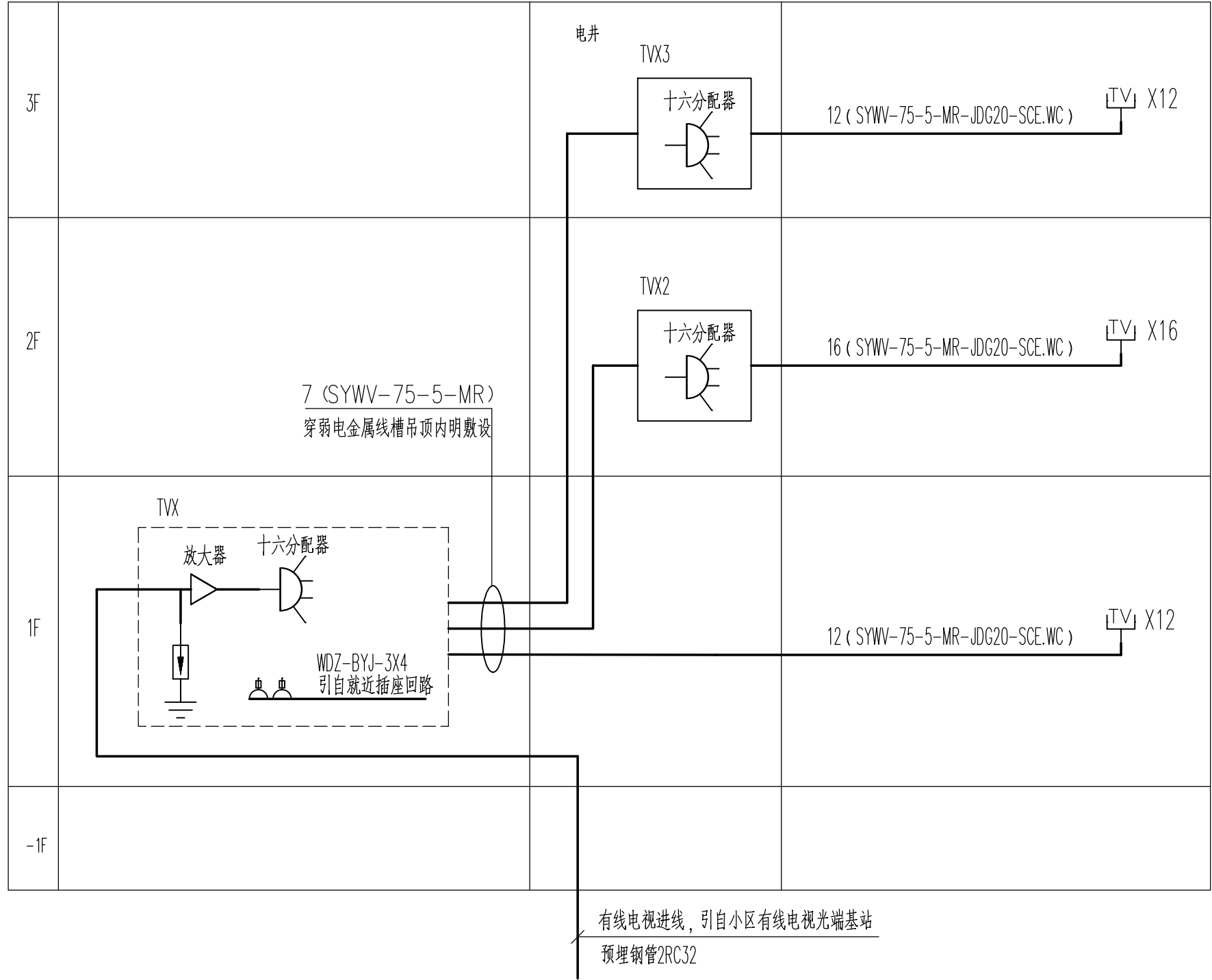
有线电视系统图
