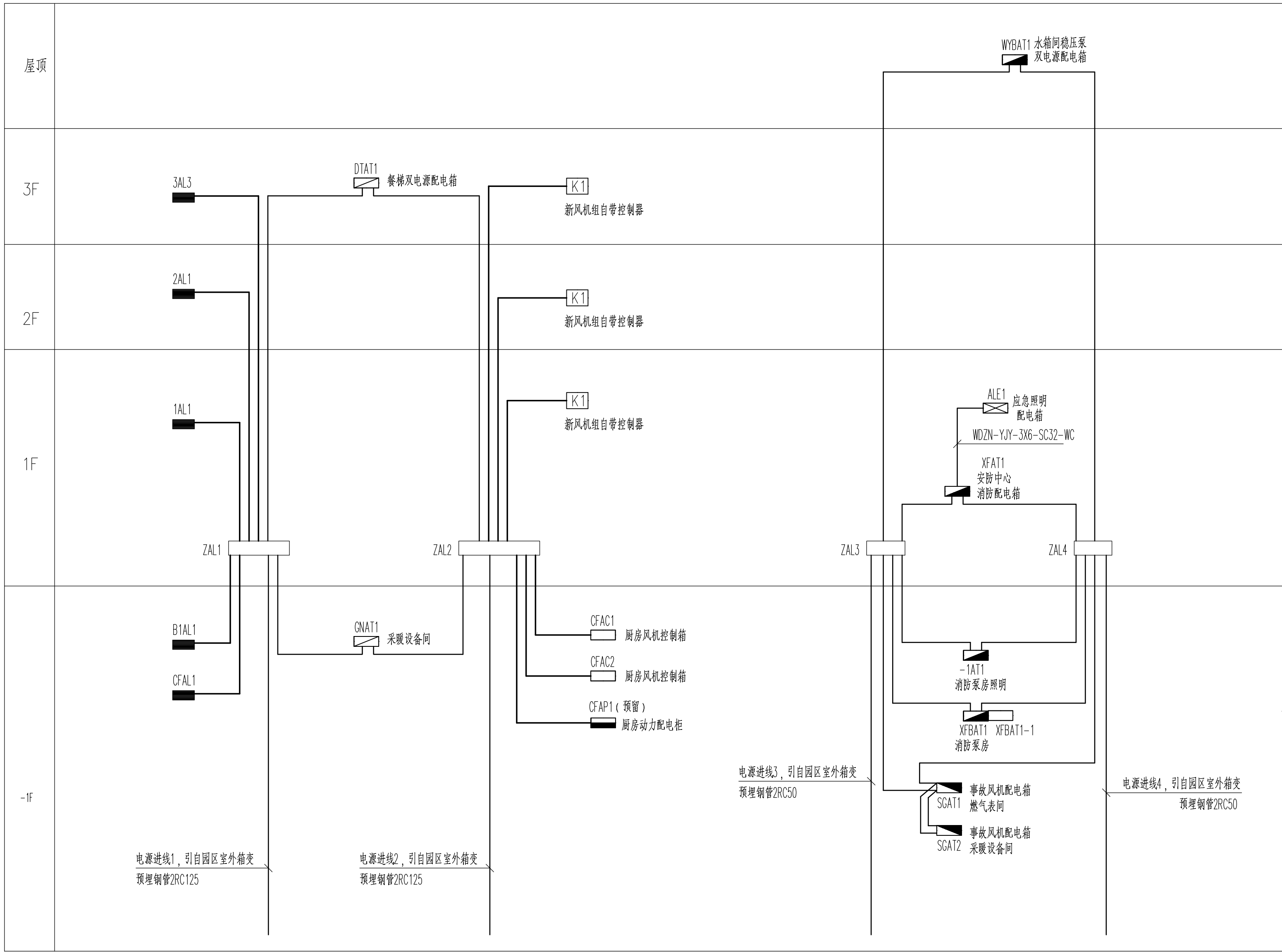
配电干线系统图
