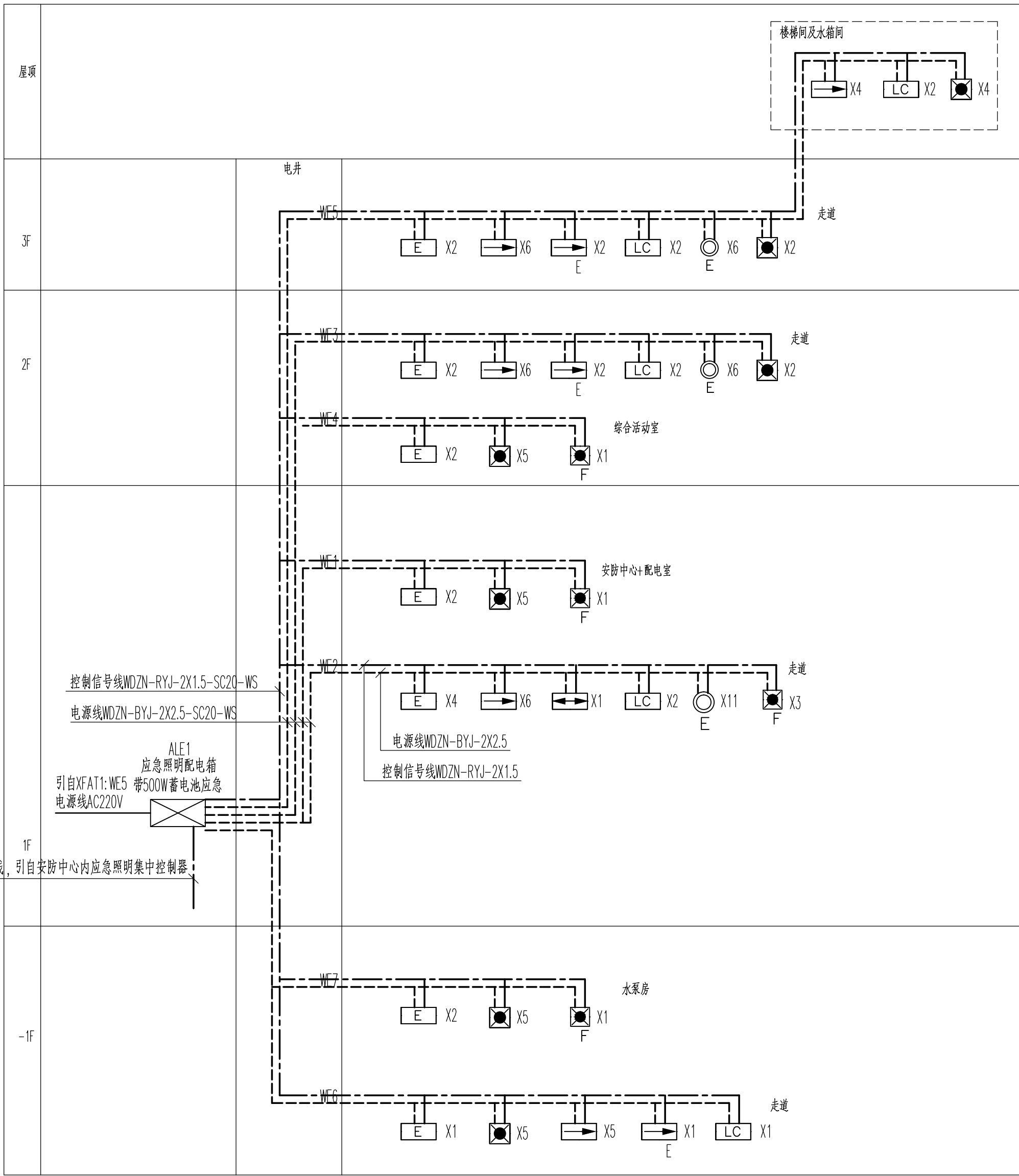
应急照明系统图
