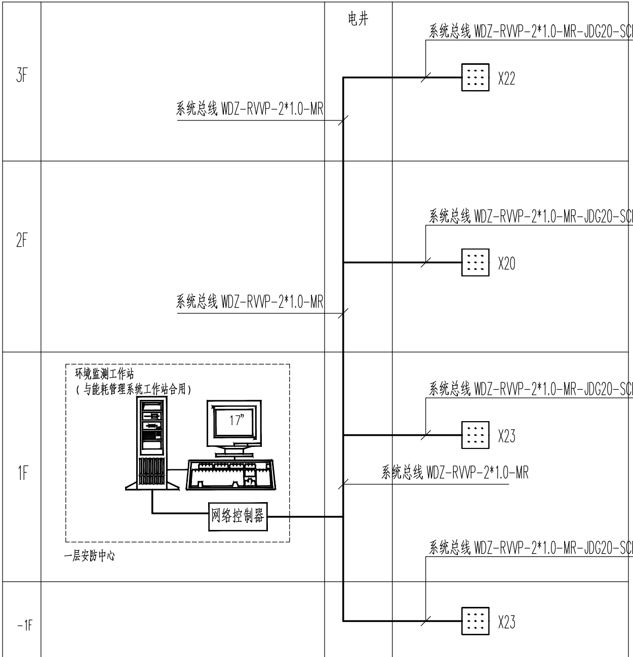
环境监测系统图
