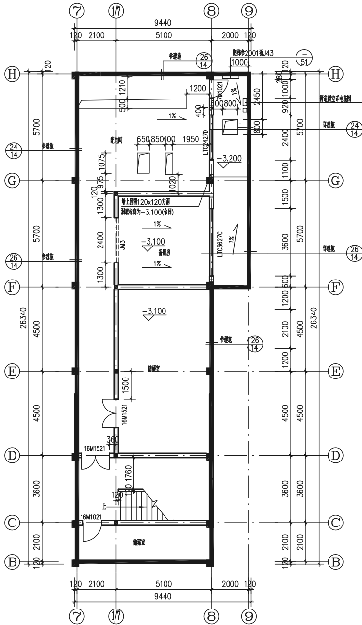
半地下室-3.100标高平面 1:100
