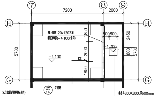
半地下室-4.100标高平面 1:100
