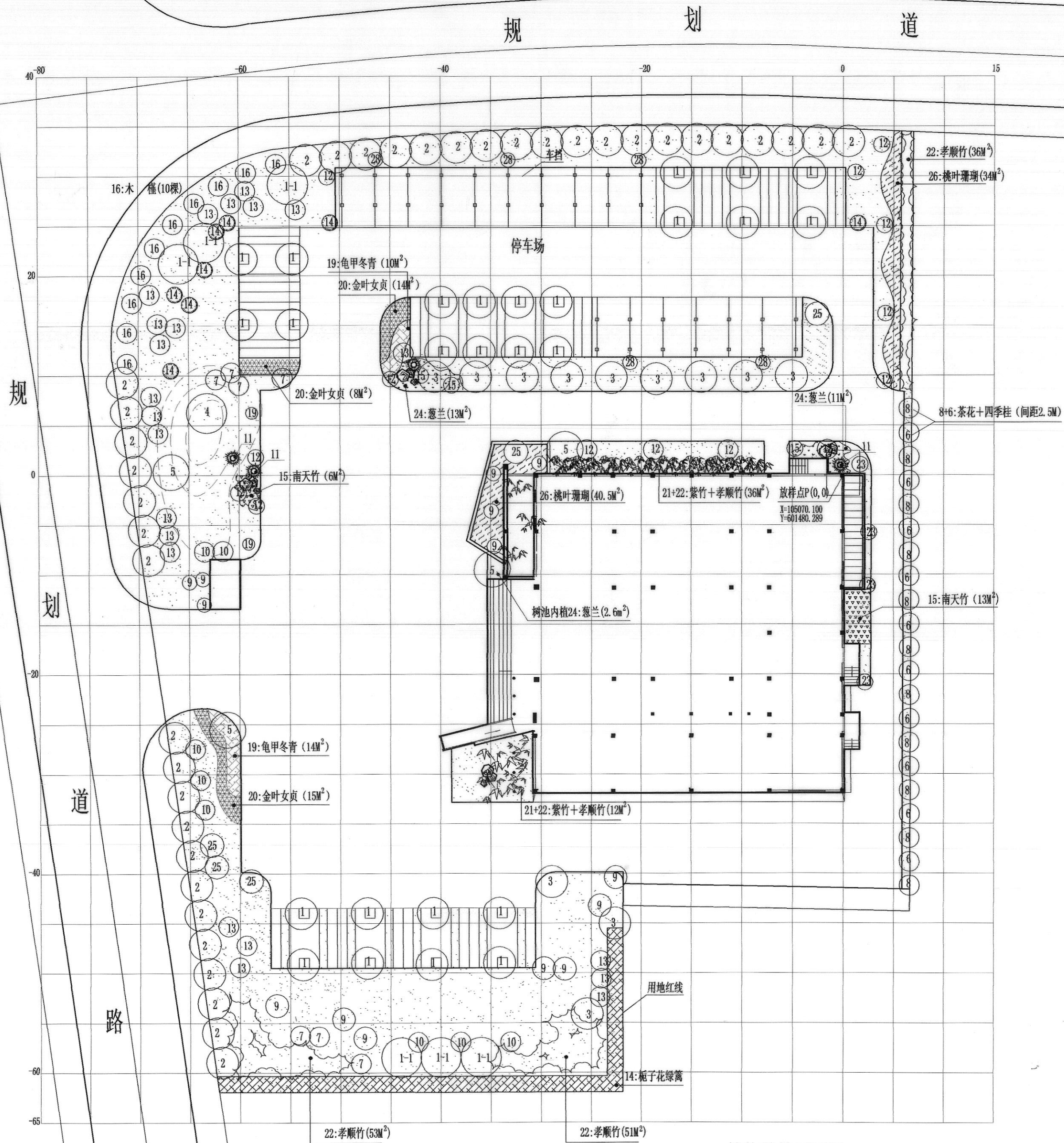
植物种植平面图 1:300
