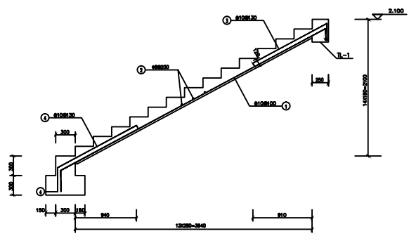
TB-1 1:25
