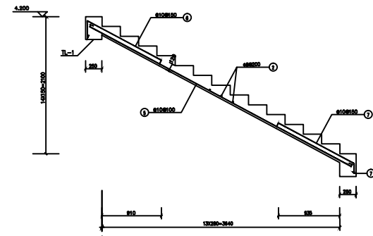
TB-2 1:25
