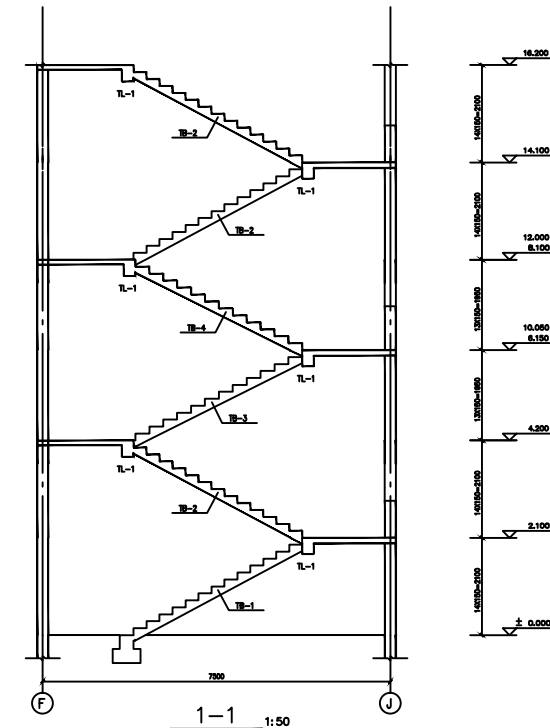
1-1 1:50
