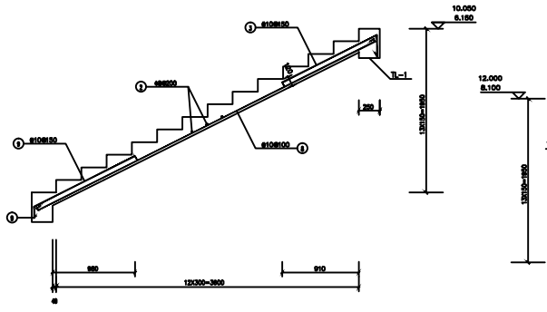
TB-3 1:25
