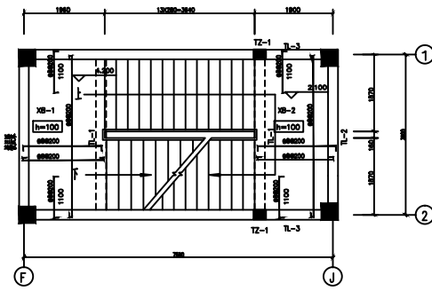
一层平面 1:50
