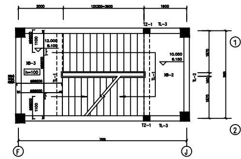
二—三层平面 1:50
