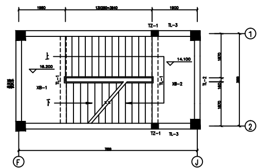
四层平面 1:50
