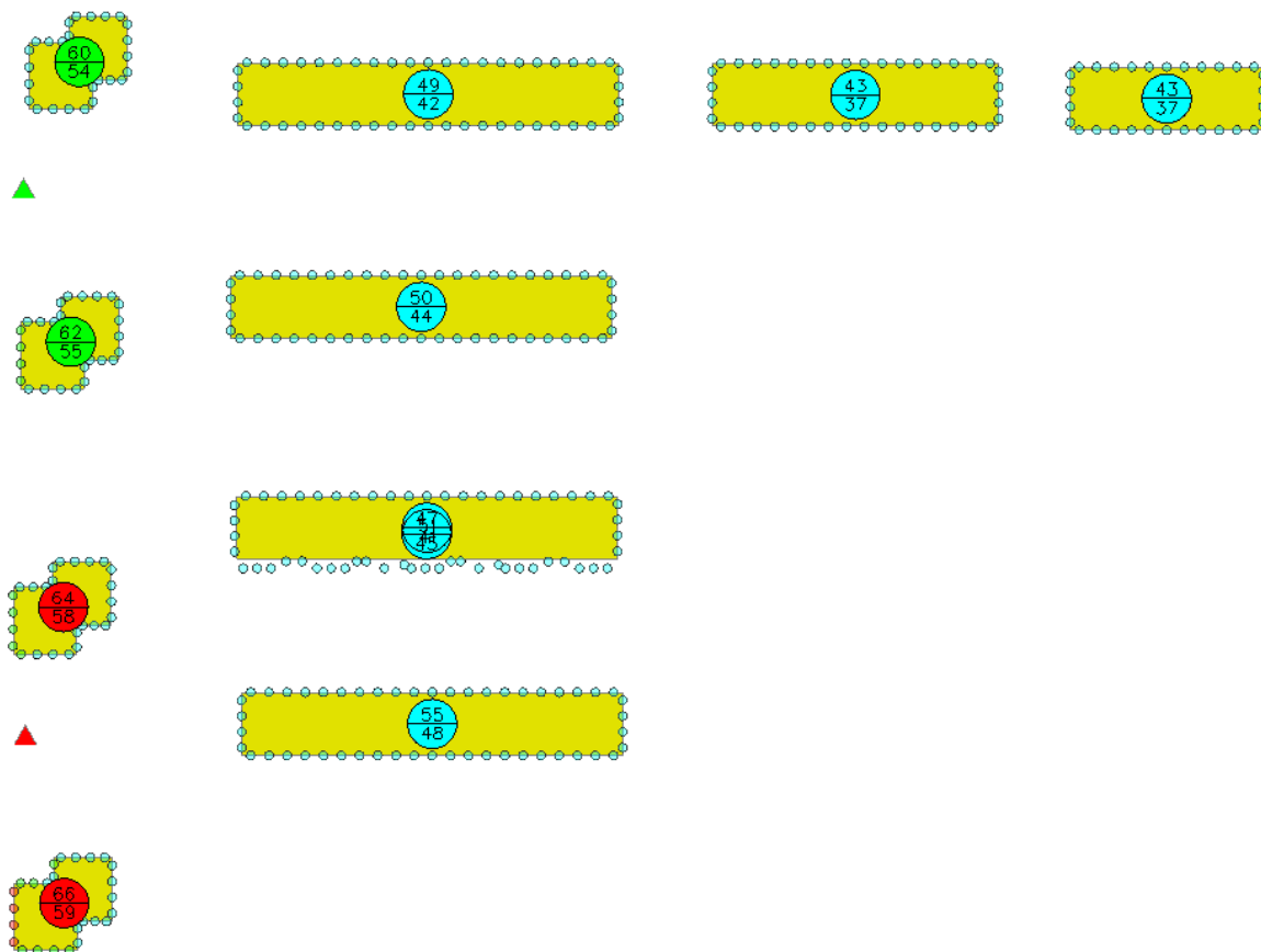
图 4.2-1 参评建筑附近区域 1.5m 高度处声压级平面分布图（昼间）
