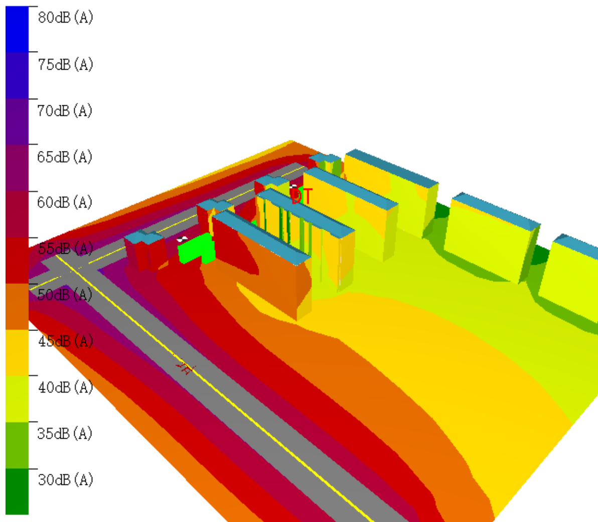
图 4.1-4 场地噪声分布俯瞰图（夜间）
