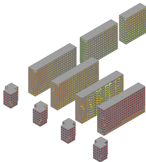
图 4.2-3 参评建筑附近区域声压级鸟瞰分布图（昼间）
