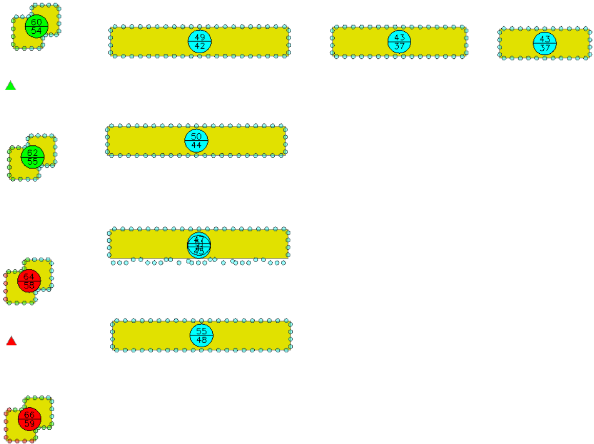
图 4.2-2 参评建筑附近区域 1.5m 高度处声压级平面分布图（夜间）
