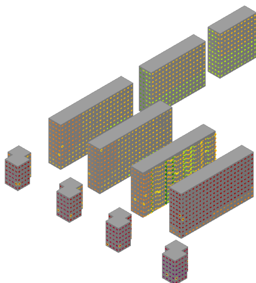
图 4.2-4 参评建筑附近区域声压级鸟瞰分布图（夜间）
