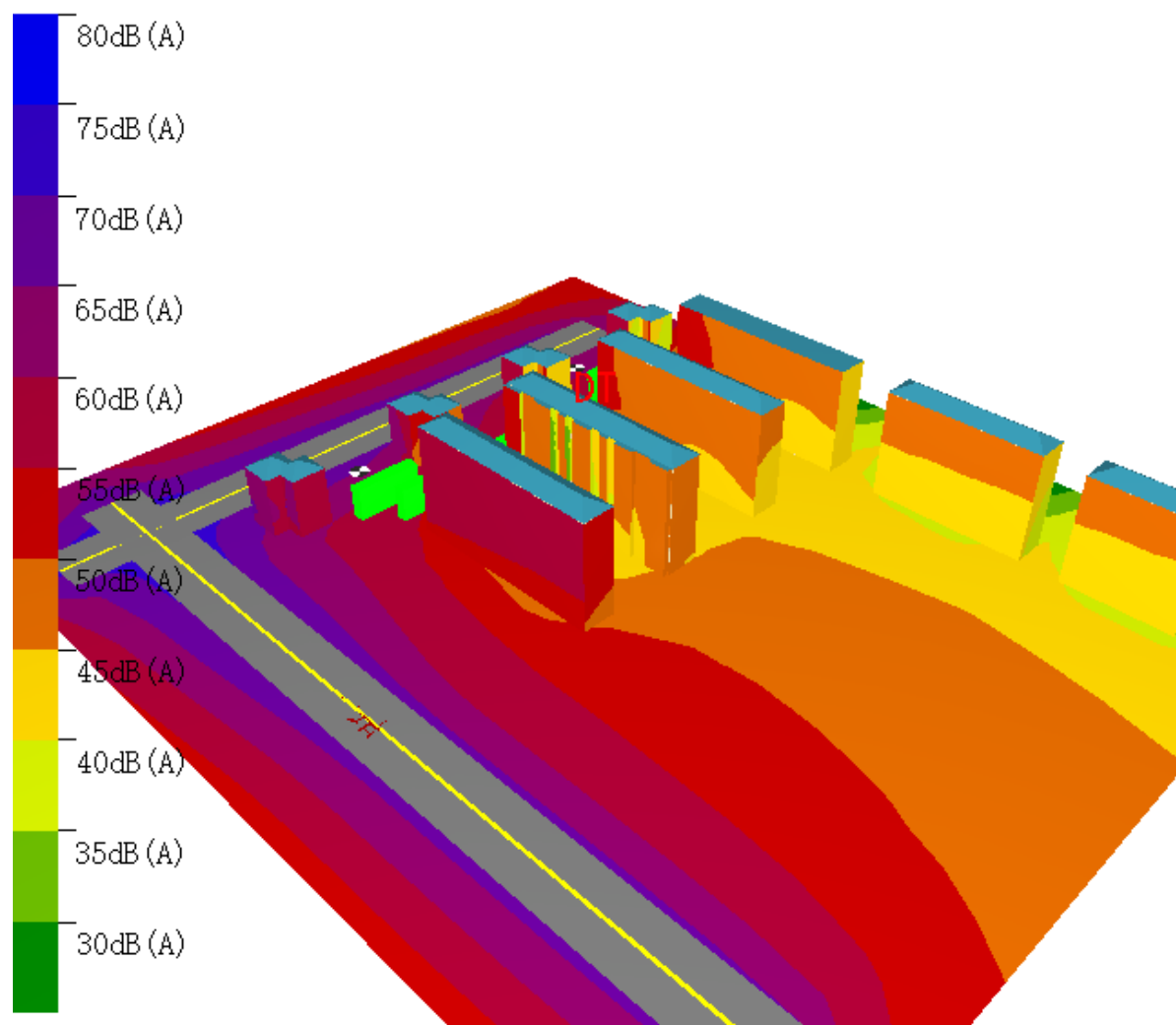
图 4.1-3 场地噪声分布俯瞰图（昼间）
