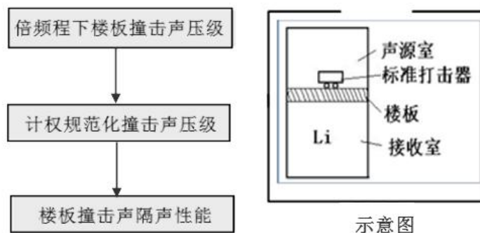
图 6-1 楼板撞击声隔声性能计算过程及测量示意图
