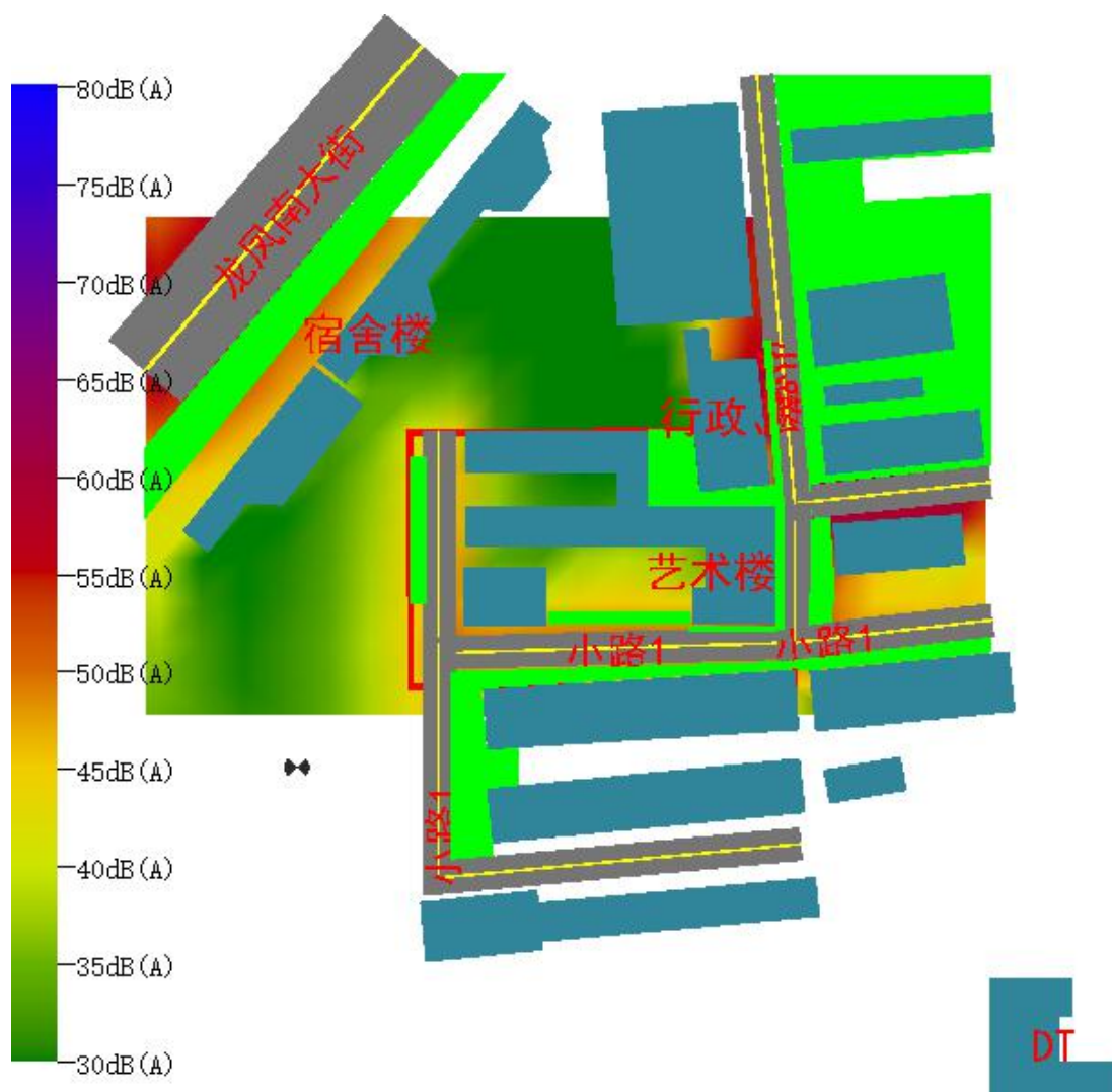
图 4.1-2 场地 1.5m 高度处声压级分布图（夜间）
