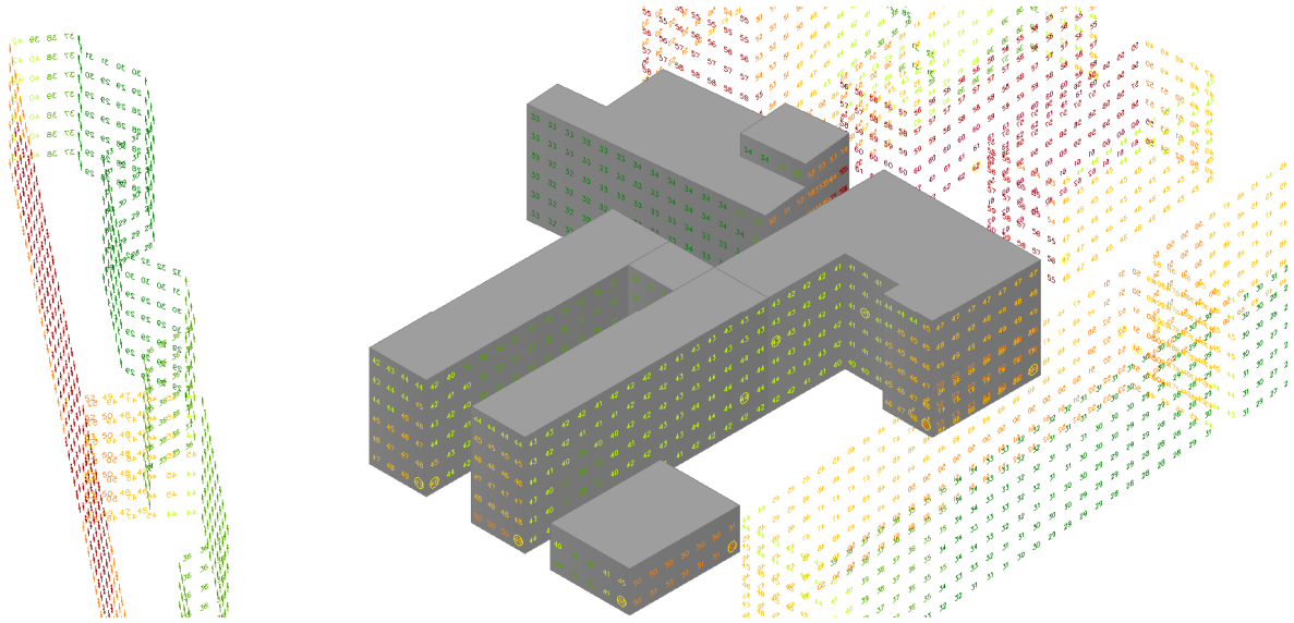
图 4.2-3 参评建筑附近区域声压级鸟瞰分布图（昼间）
