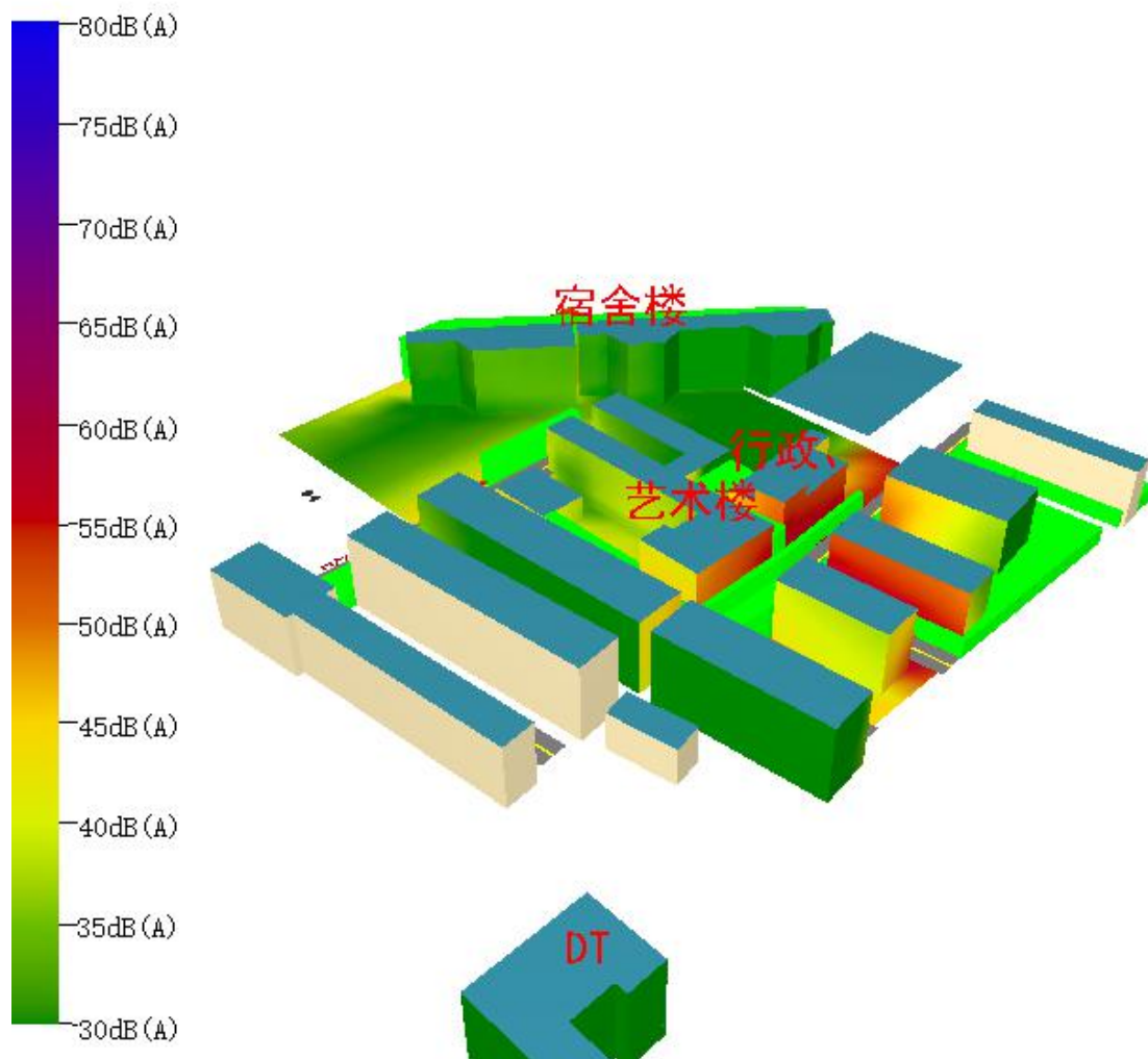
图 4.1-4 场地噪声分布俯瞰图（夜间）
