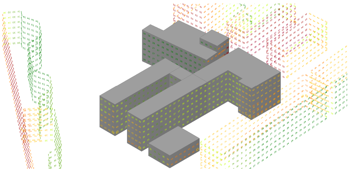
图 4.2-4 参评建筑附近区域声压级鸟瞰分布图（夜间）
