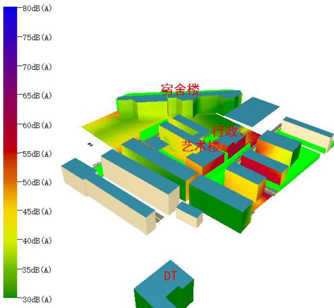
图 4.1-3 场地噪声分布俯瞰图（昼间）
