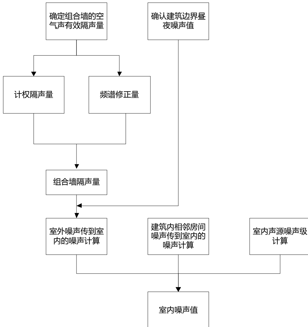
图 5.2-2 室内噪声计算原理图
