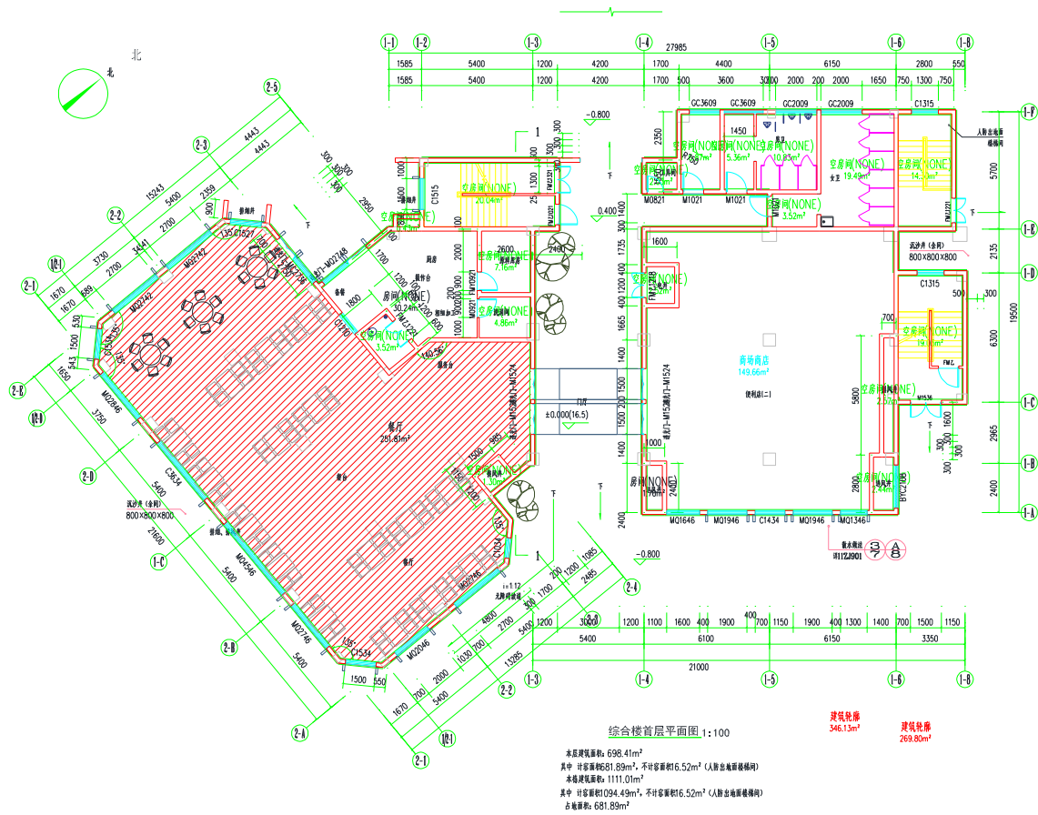
图 7-1 最不利房间楼层平面图
