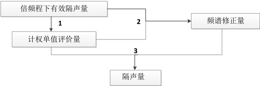
图 7.4-1 组合墙空气声隔声量计算原理图
