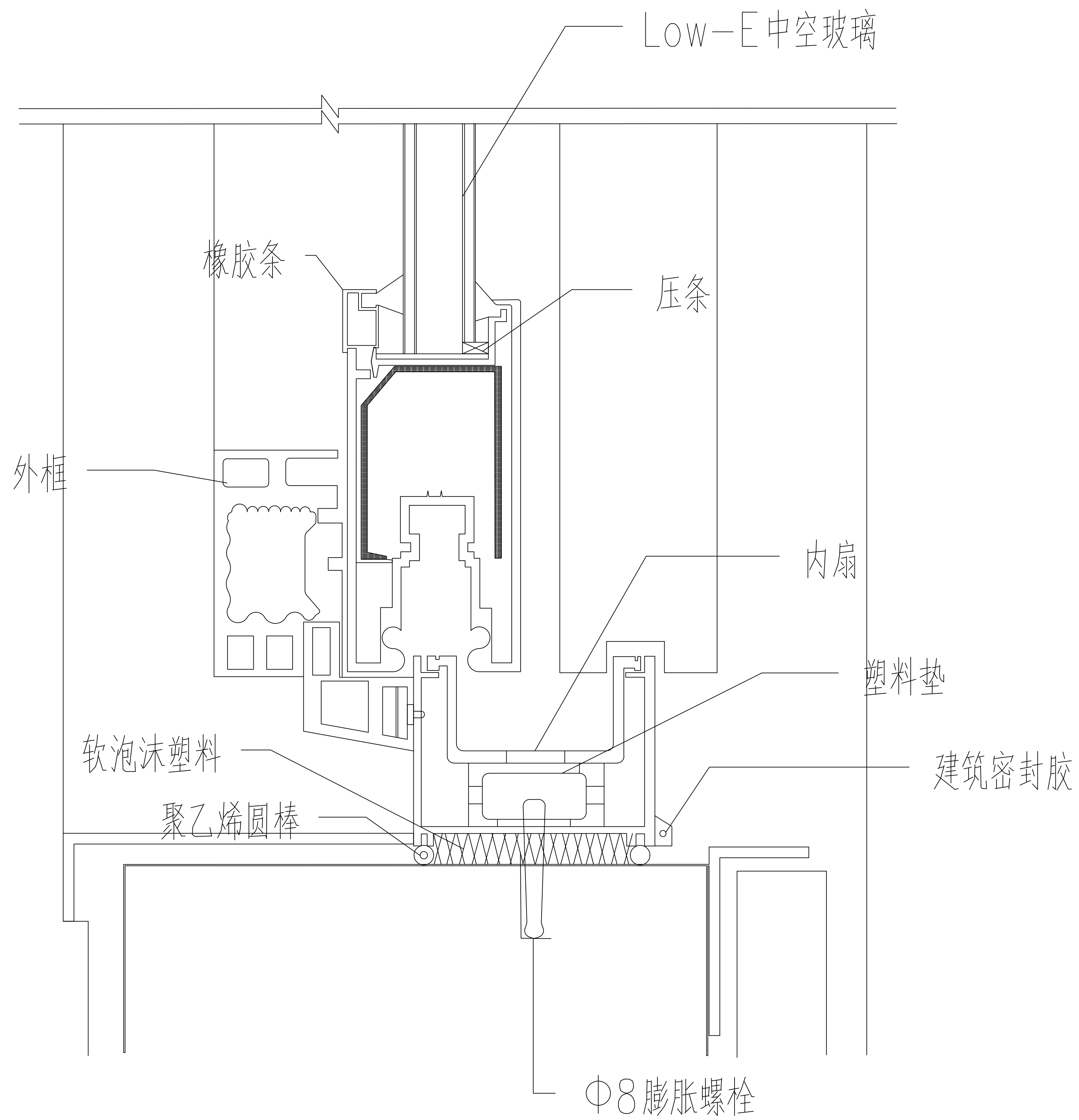
塑钢门窗构造
