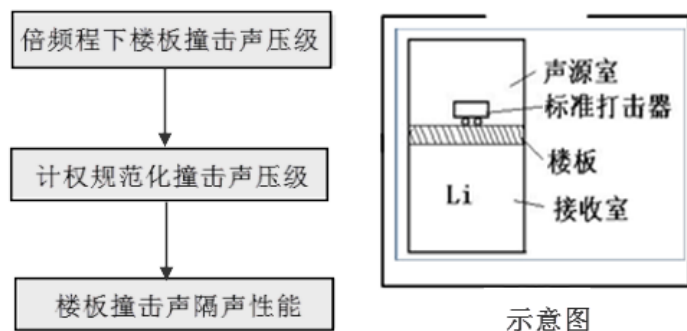
图 6-1 楼板撞击声隔声性能计算过程及测量示意图
