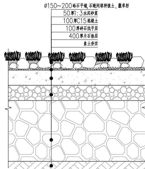
5 卵石嵌铺路面做法 SCALE 1:10
