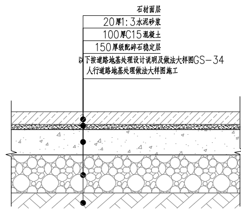
2 人行道石材路面做法 SCALE 1:10
