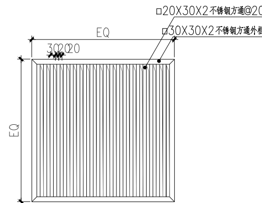
10 泵坑钢格栅平面图 SCALE 1:10
