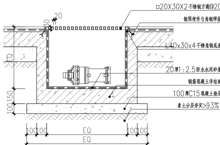
9 石材池底池壁做法 SCALE 1:15
