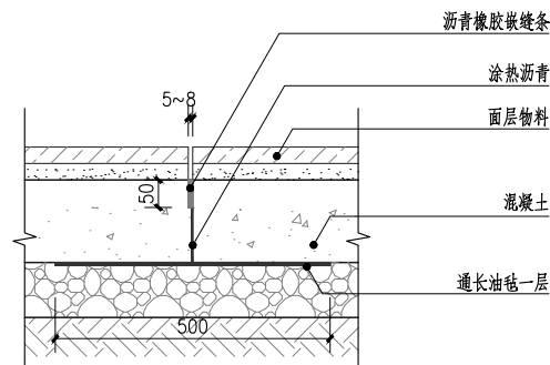
6 广场及道路缩(纵)缝大样图 SCALE 1:10
