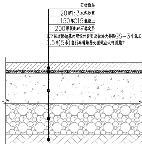
1 广场石材路面做法 SCALE 1:10
