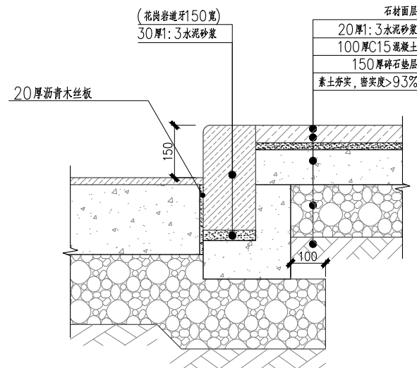
4 立道牙做法五 SCALE 1:10
