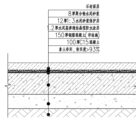
3 水池底(壁)构造 SCALE 1:20
