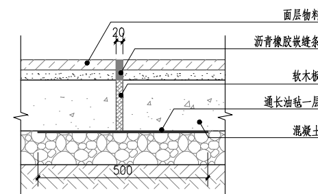
7 广场及道路胀缝大样图 SCALE 1:10
