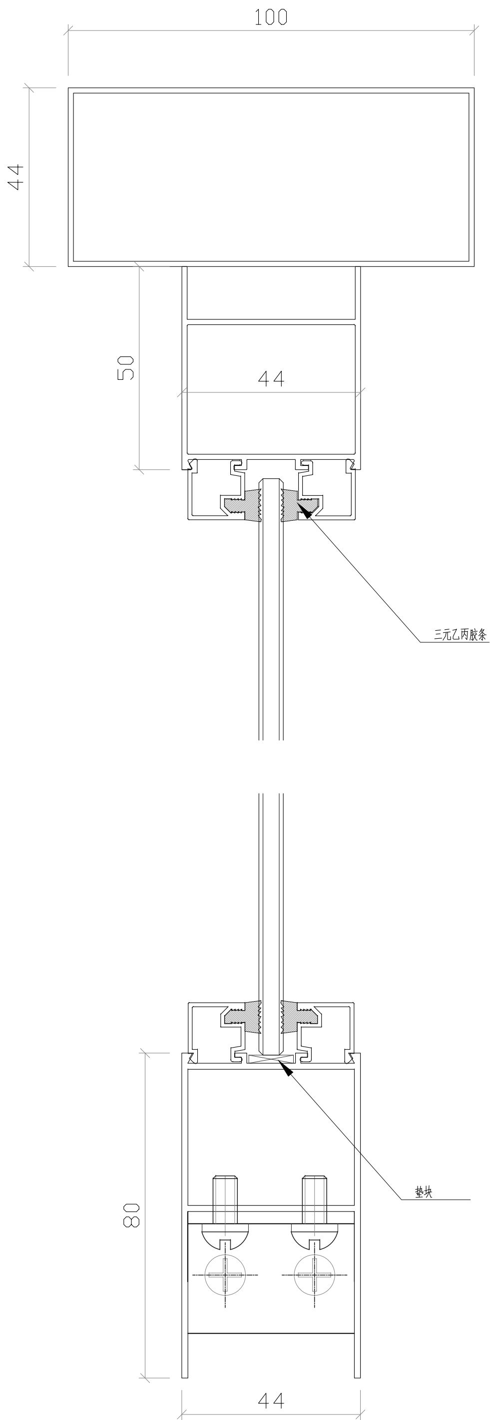
铝合金门纵剖节点图 1:1
