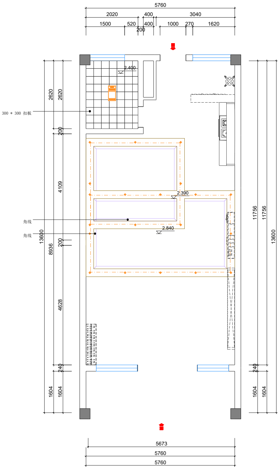
综合天花(1:90)
