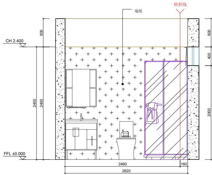
卫生间立面D(1:50)
