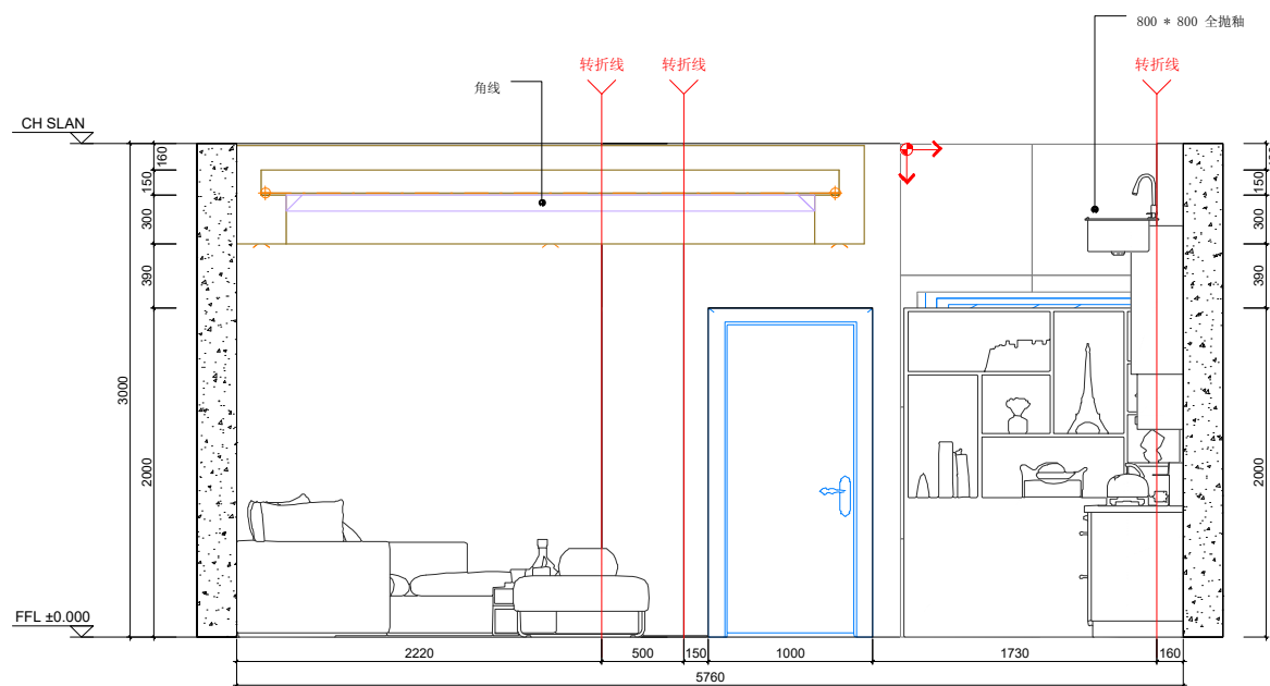
客餐厅立面A(1:50)
