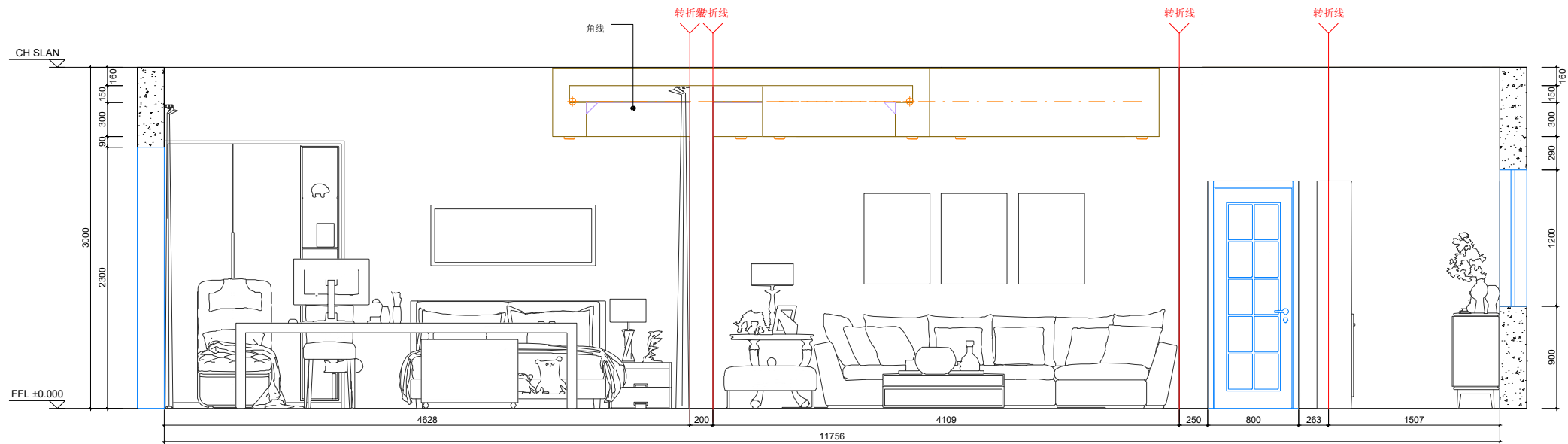
客餐厅立面D(1:50)
