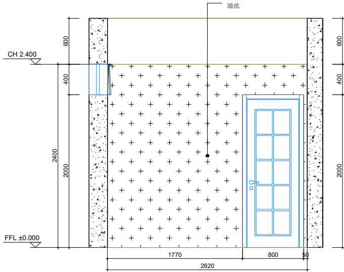
卫生间立面B(1:50)
