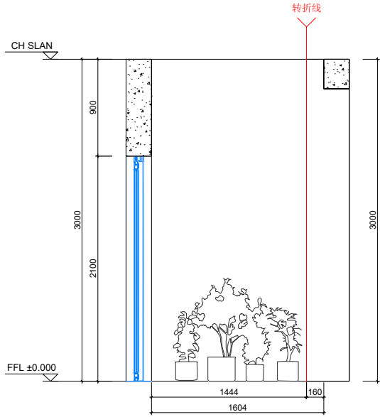
阳台立面B(1:50)
