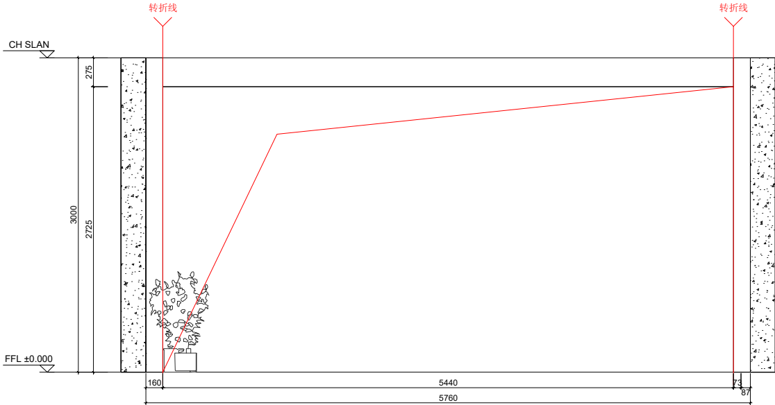
阳台立面C(1:50)
