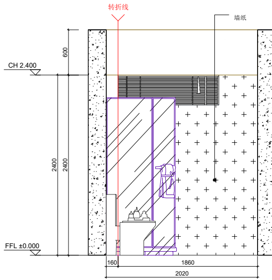
卫生间立面A(1:50)
