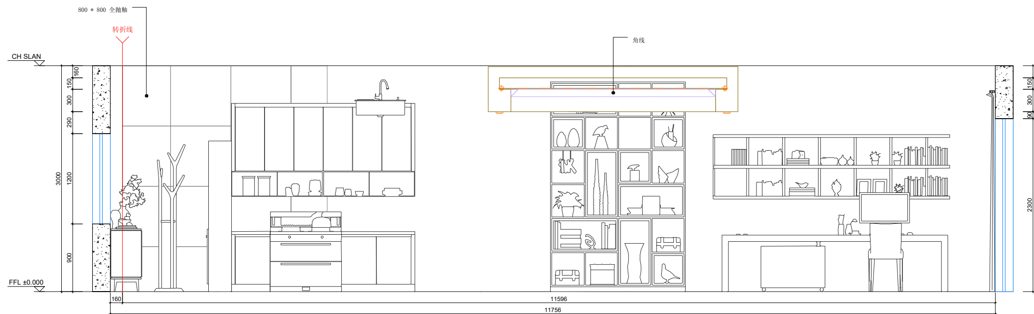
客餐厅立面B(1:50)
