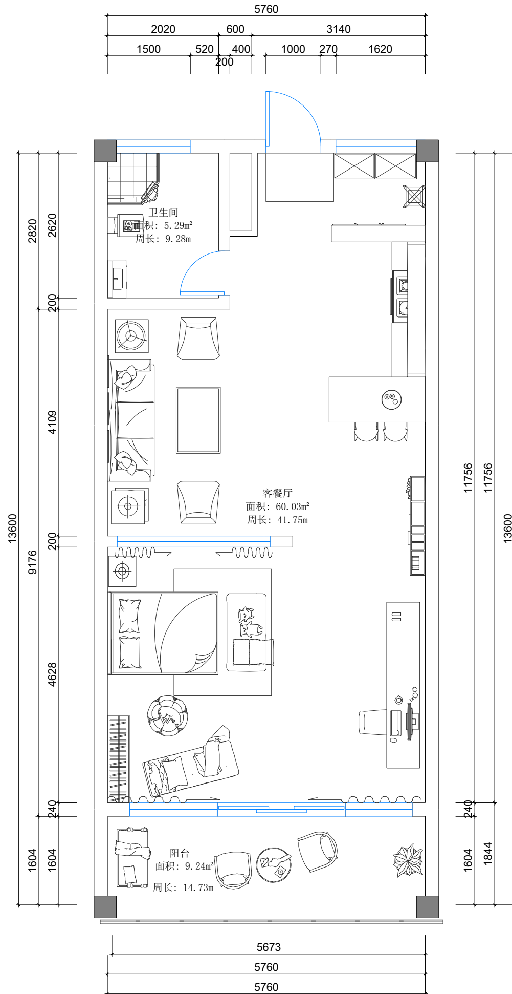
平面布置(1:70)
