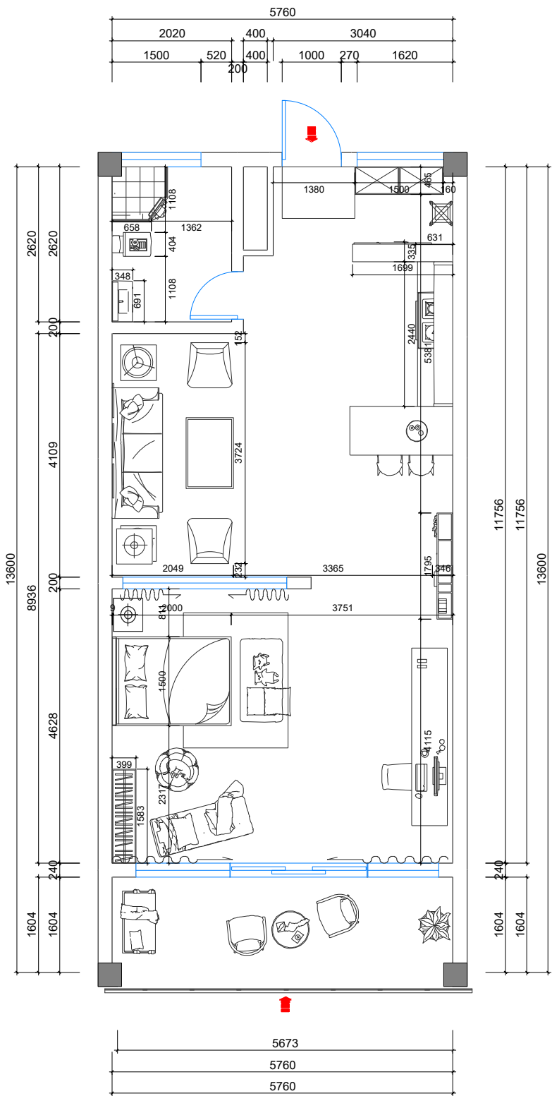
家具尺寸(1:90)
