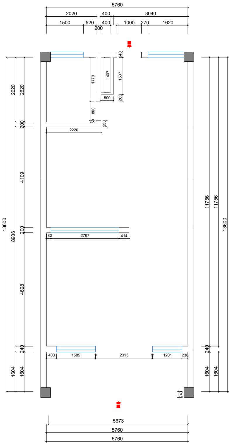
墙体定位(1:90)
