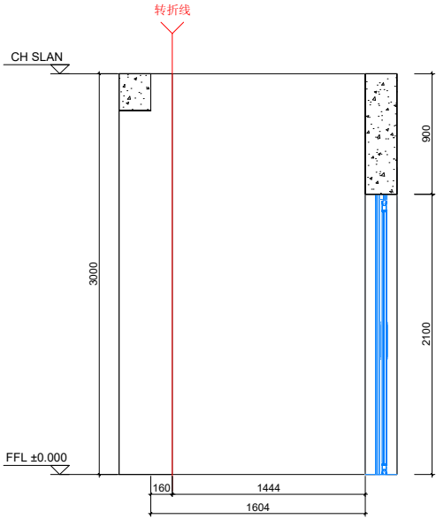
阳台立面D(1:50)
