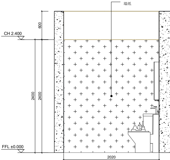
卫生间立面C(1:50)
