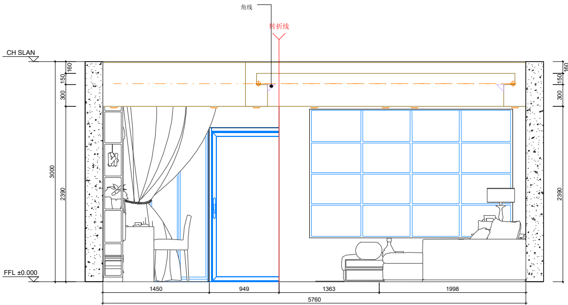
客餐厅立面C(1:50)
