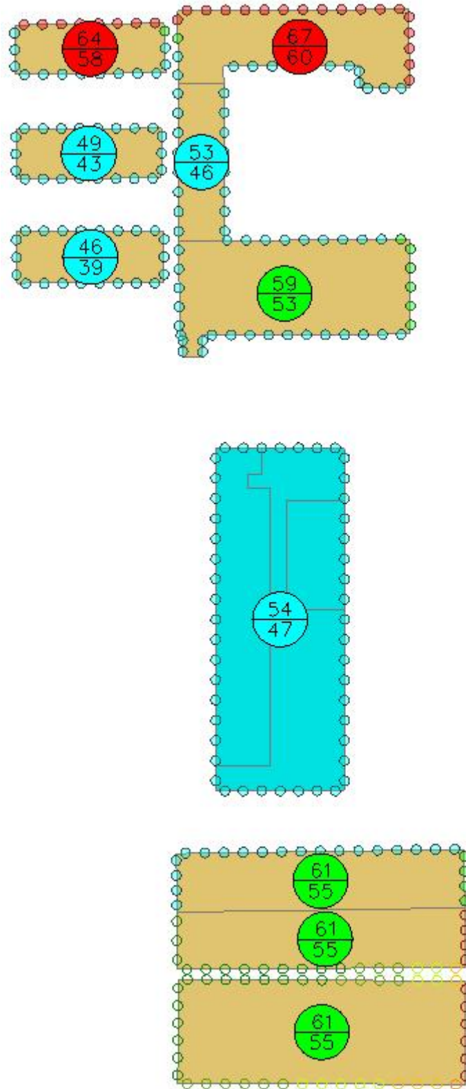
图 4.2-2 参评建筑附近区域 1.5m 高度处声压级平面分布图（夜间）
