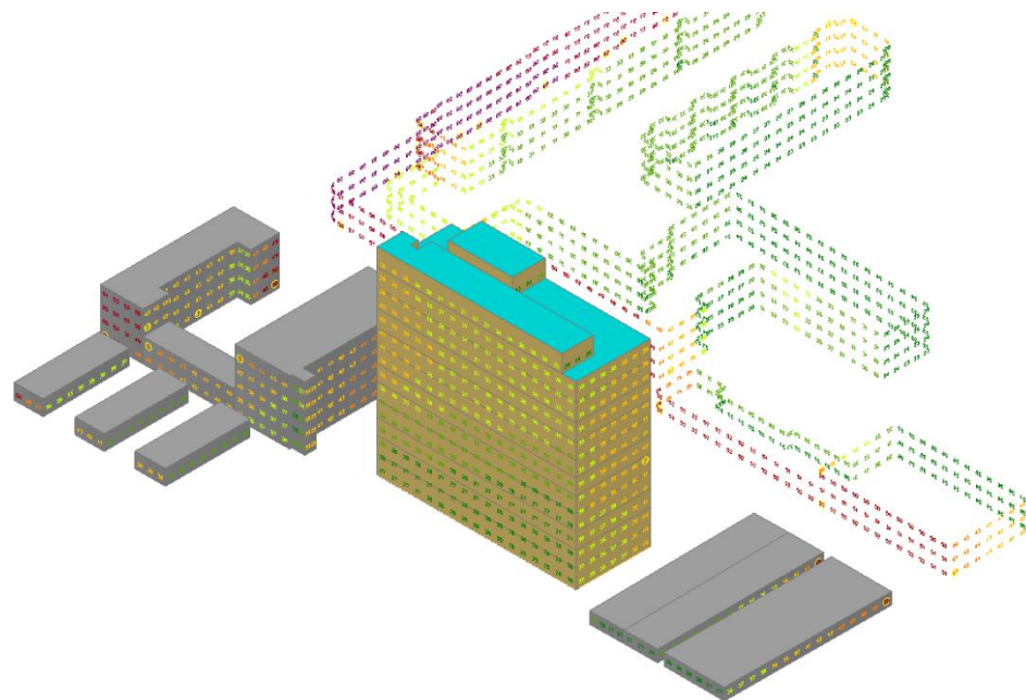
图 4.2-4 参评建筑附近区域声压级鸟瞰分布图（夜间）
