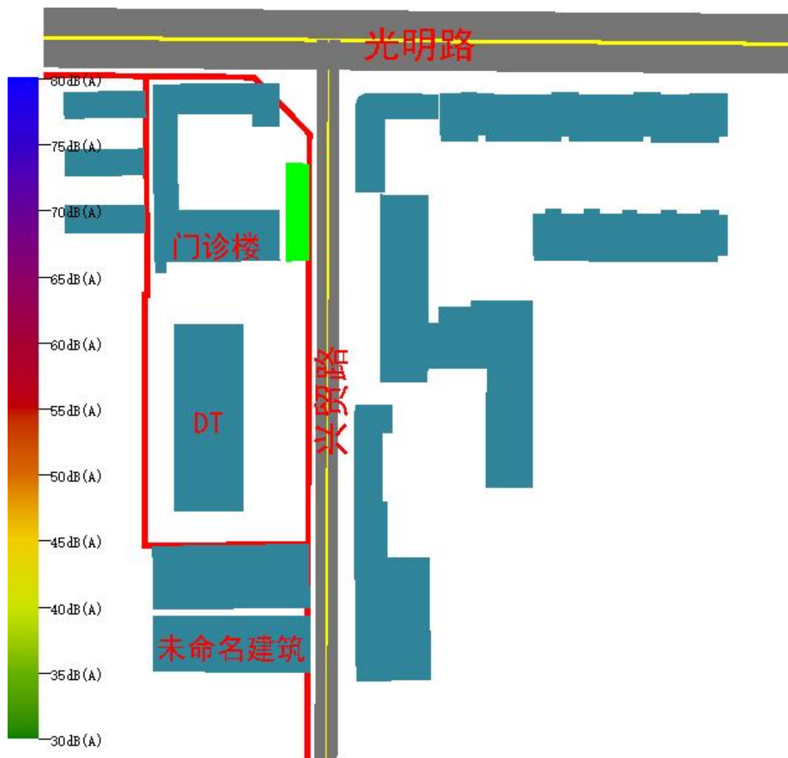
图 4.1-2 场地 1.5m 高度处声压级分布图（夜间）
