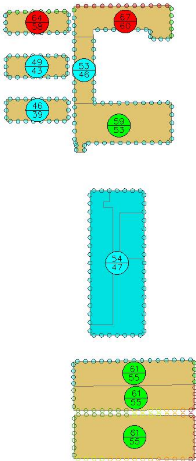
图 4.2-1 参评建筑附近区域 1.5m 高度处声压级平面分布图（昼间）
